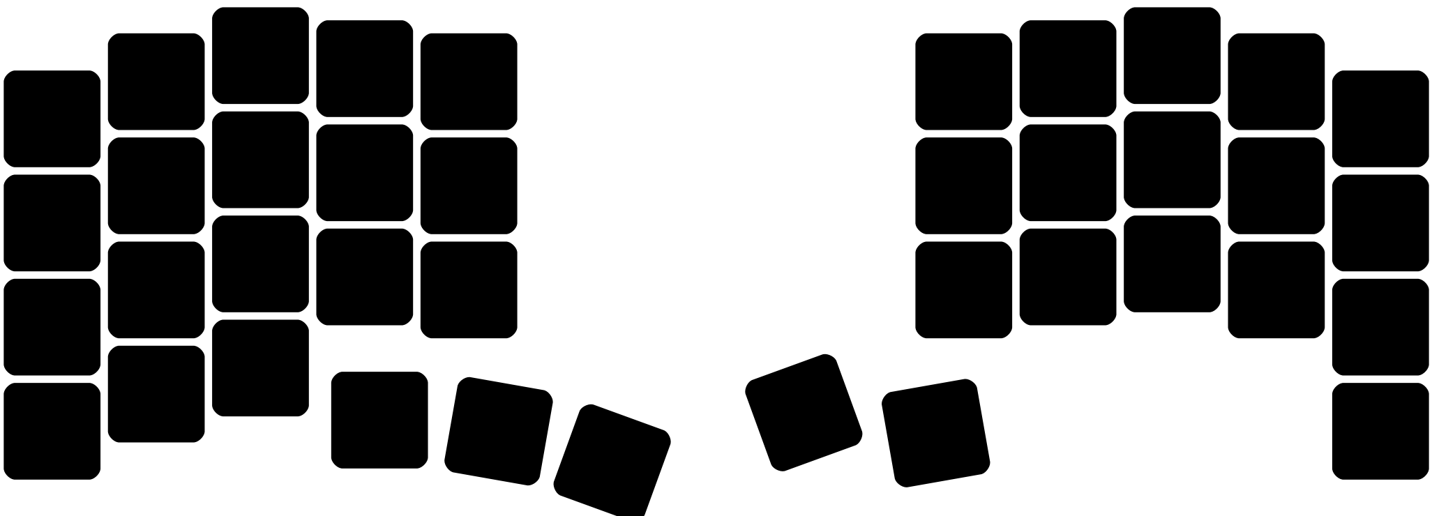
Emacs:
