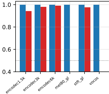
detection AUC
