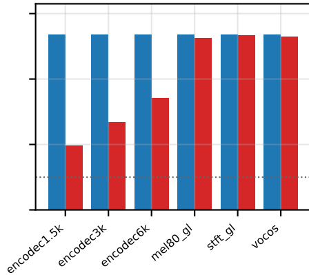
invariant_ss
