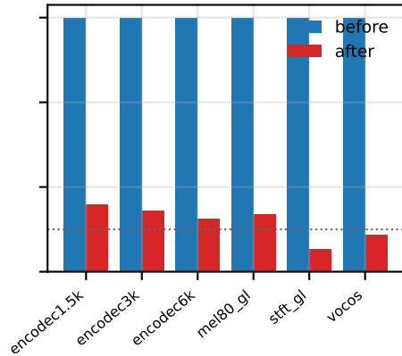
surface_ss
