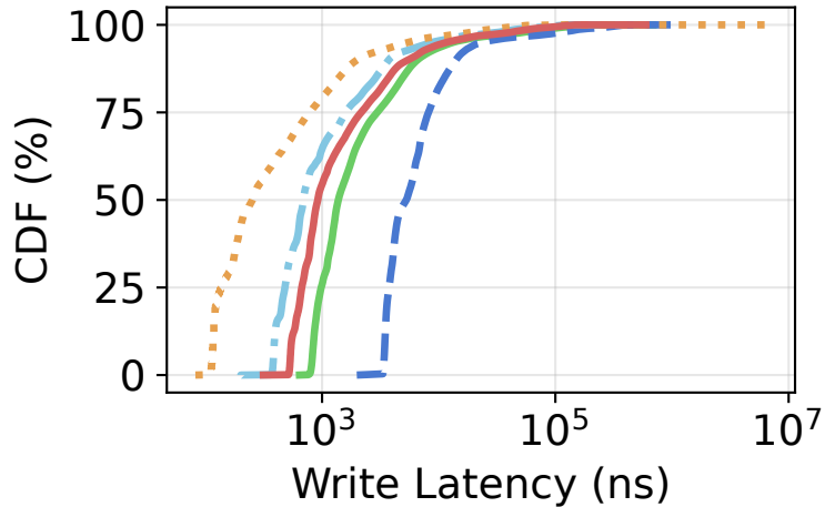
Online Boutique
