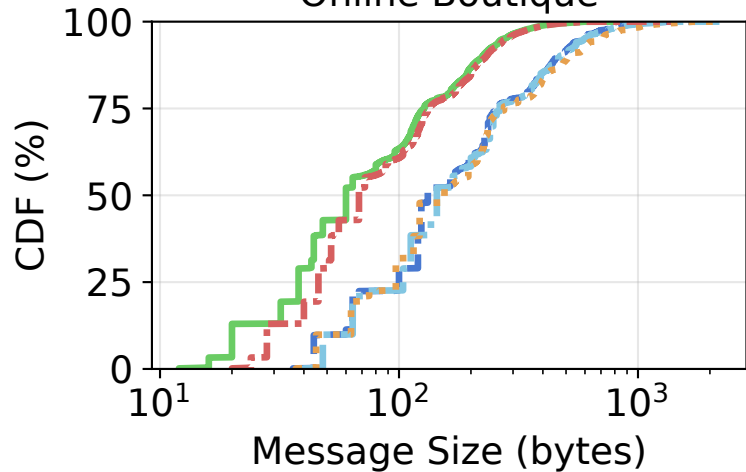
Online Boutique
