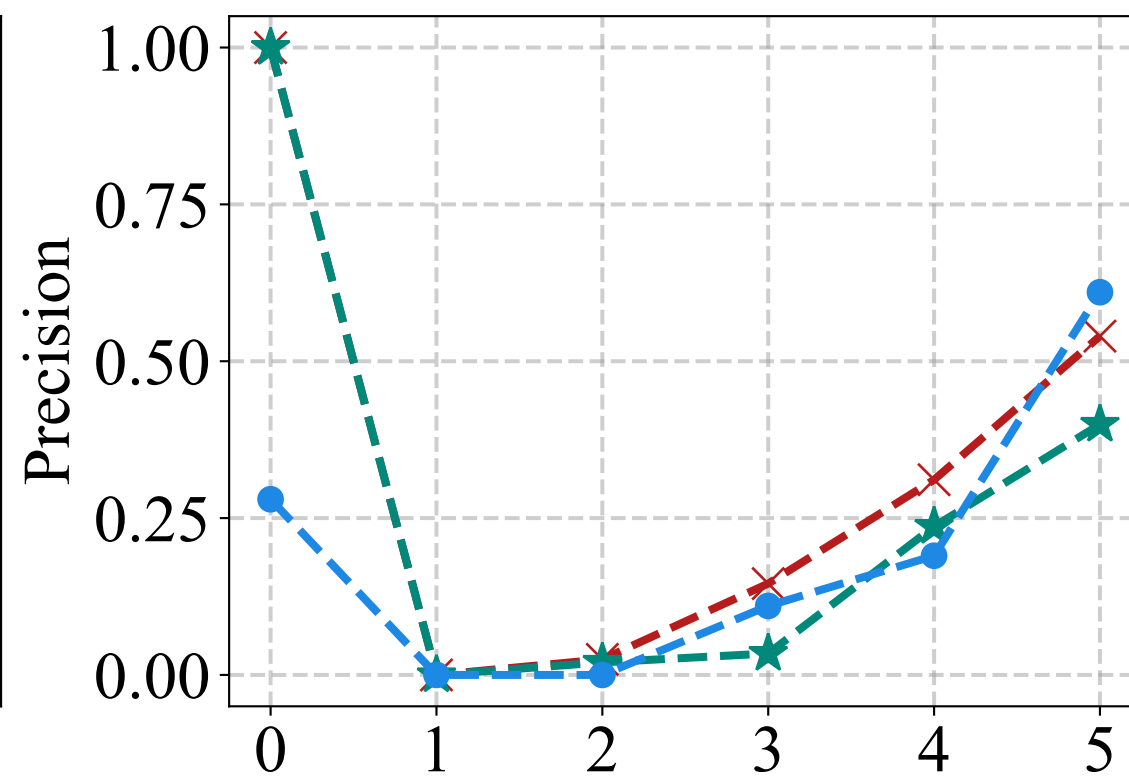
Zero-shot: Precision
