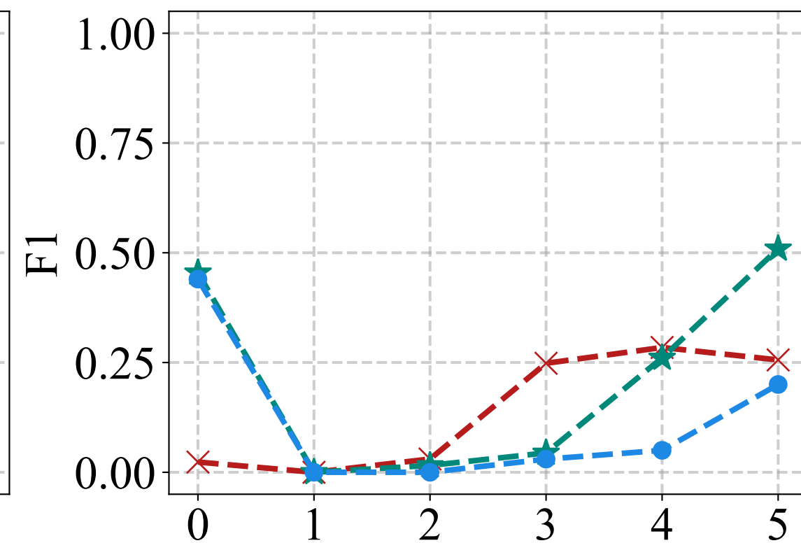
Zero-shot: F1
