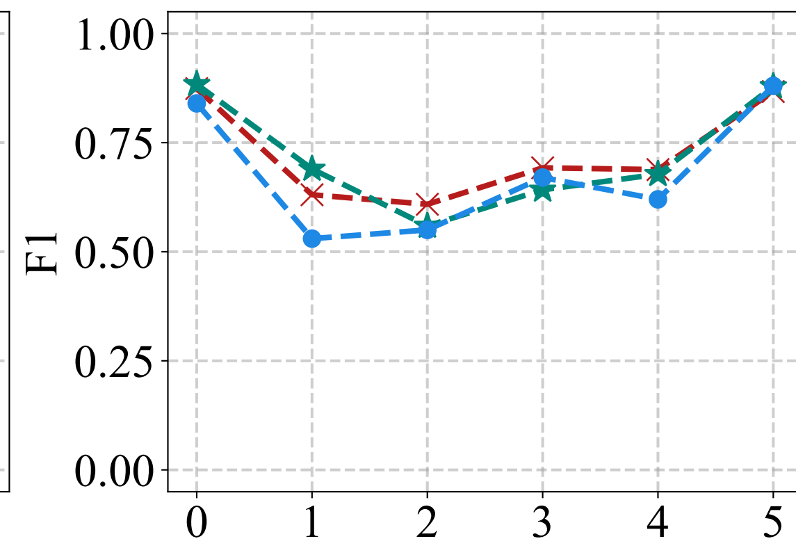
Fine-tuned: F1
