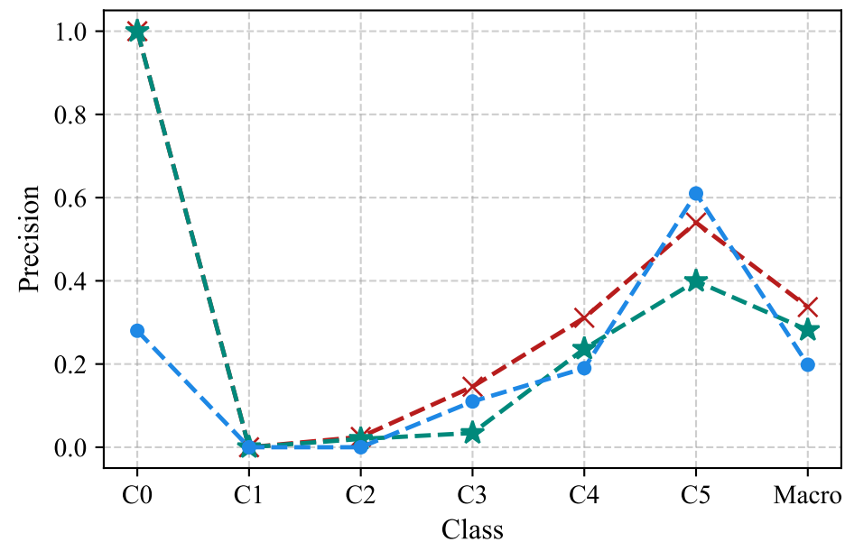
Zero-shot: Precision
