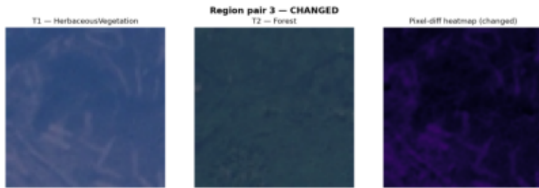
heatmap_pair_03_changed.png
