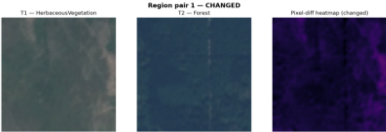
heatmap_pair_01_changed.png
