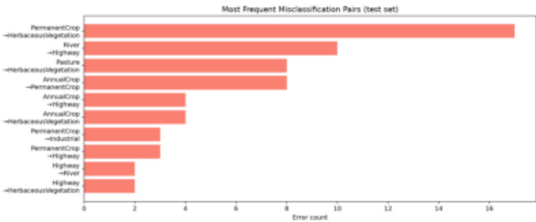
confusion_pair_chart.png
