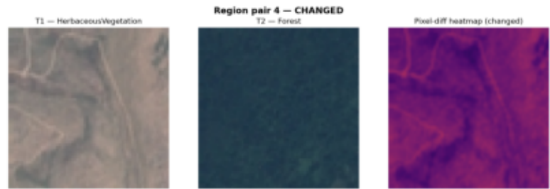
heatmap_pair_04_changed.png
