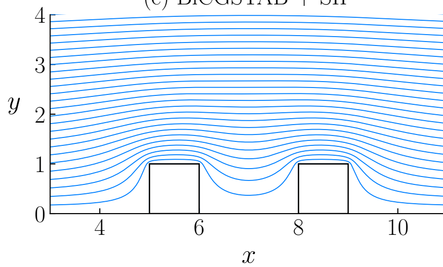
(e) BiCGSTAB + SIP
