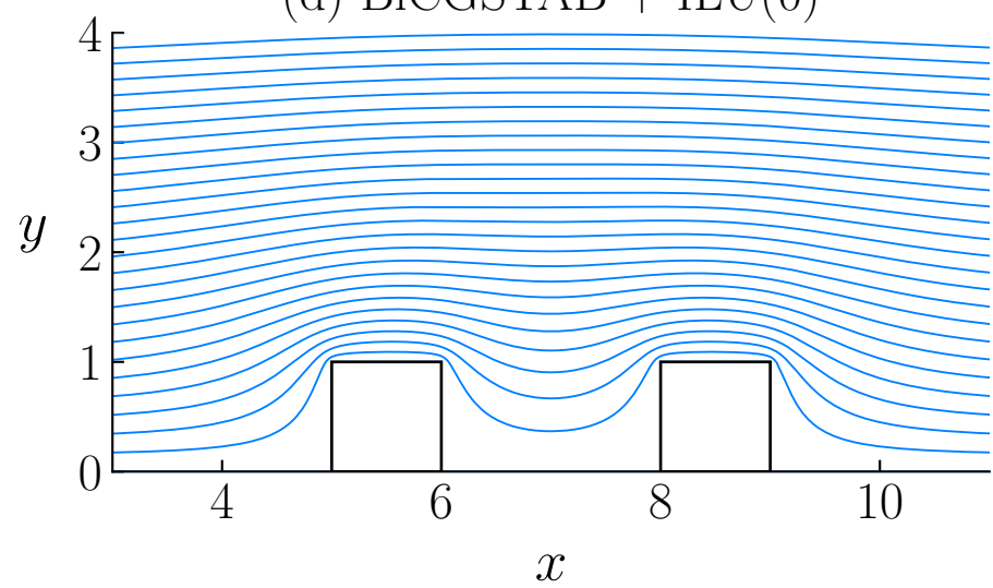
(d) BiCGSTAB + ILU(0)
