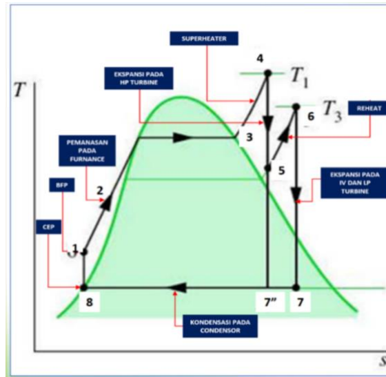
Gambar 3. 1 Konversi Energi dalam Siklus Rankine Di PLTU Paiton 9
