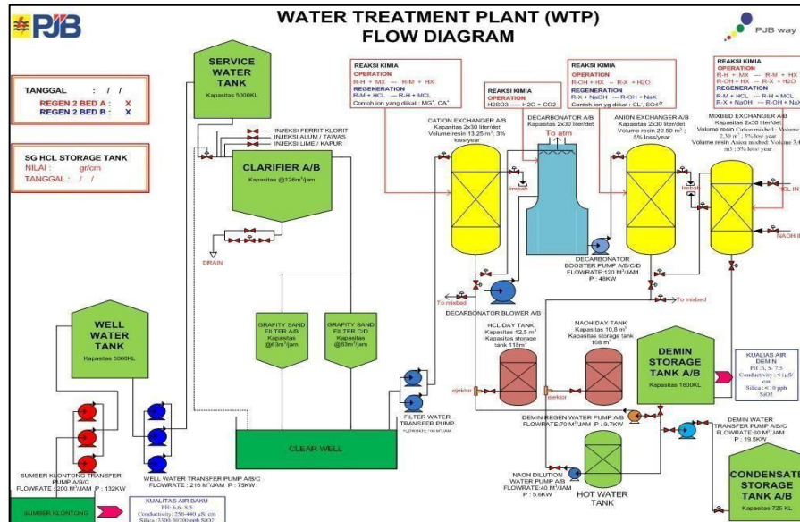
Gambar 3.11 Alur Sistem Air di PLTU
