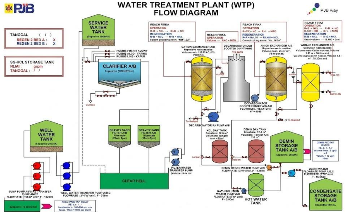
Gambar IV. 9 Diagram Alir Siklus Di WTP
