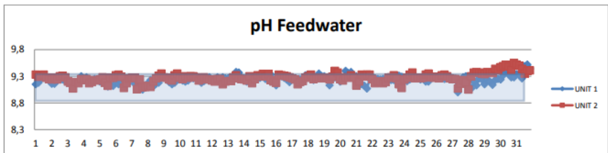
Gambar IV. 29 Grafik pH Feedwater
