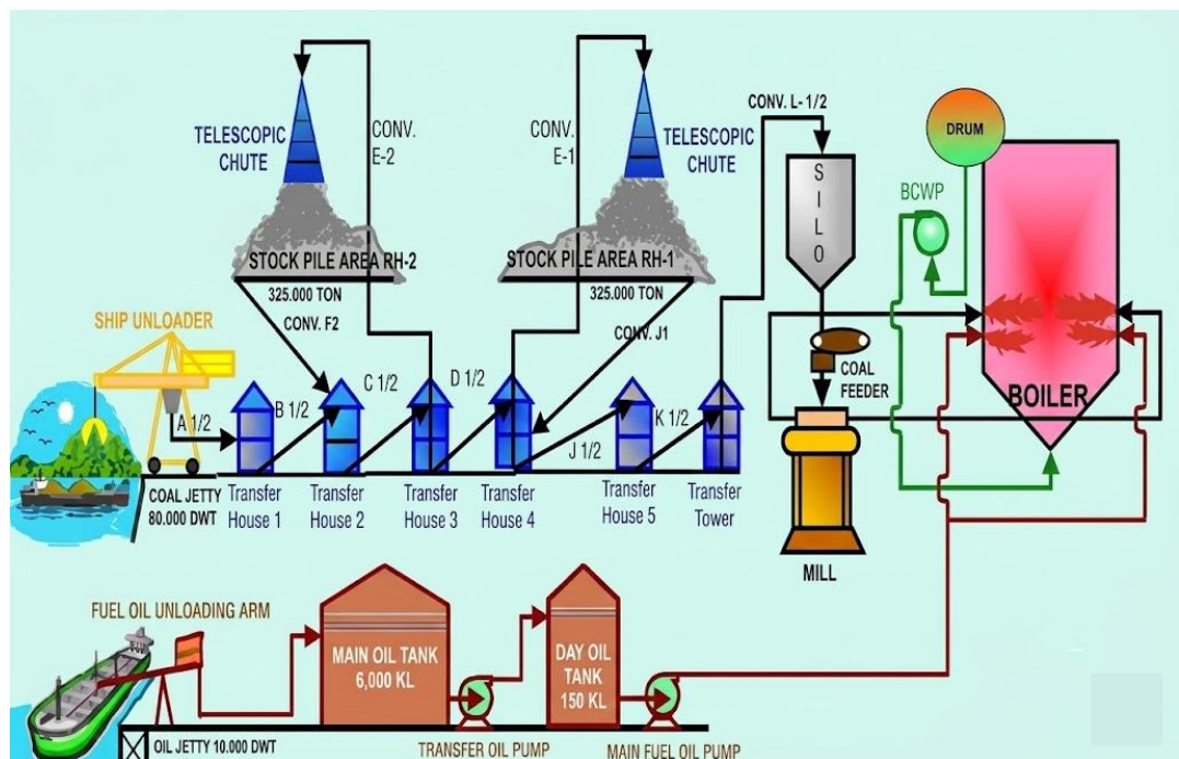
Gambar IV. 2 Sistem Bahan Bakar
