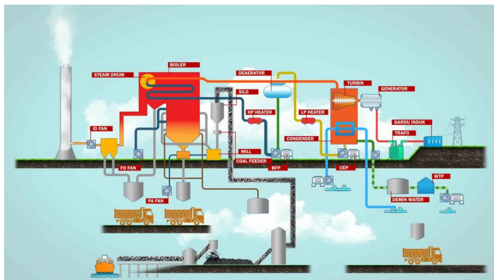
Gambar IV. 1 Alur Proses PLTU Paiton
