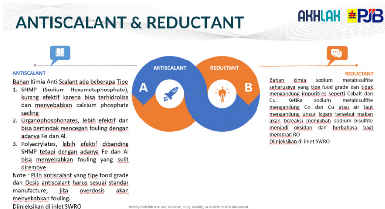
Gambar 3. 55 Antiscalant dan reductant (SWRO)
