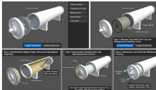
Gambar 3. 57 Simulasi Pergantian Membran Baru
