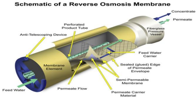
Gambar 3. 48 Gambar skematik Membran Reverse Osmosis
