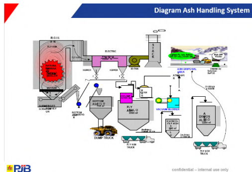
Gambar 3. 5 Sistem Penanganan Abu (Sumber : PT.PLN Nusantara Power UP Paiton)
