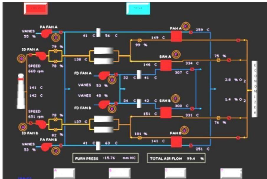
Gambar 2.8 Diagram alur udara dan flue gas
