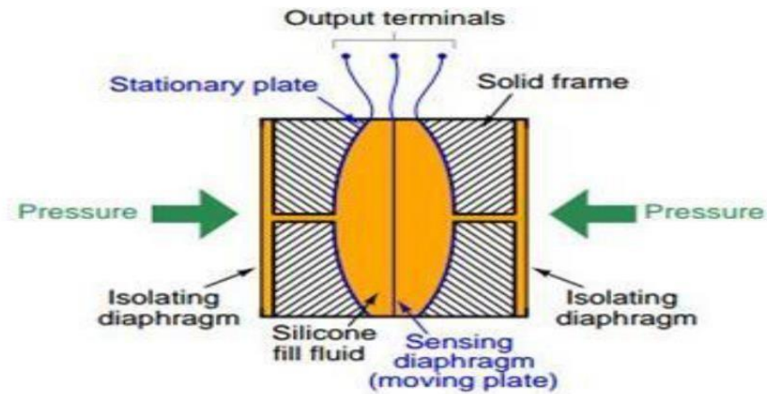
Gambar 3.6 Bagian – bagian dalam Diffrential Pressure Transmitter
