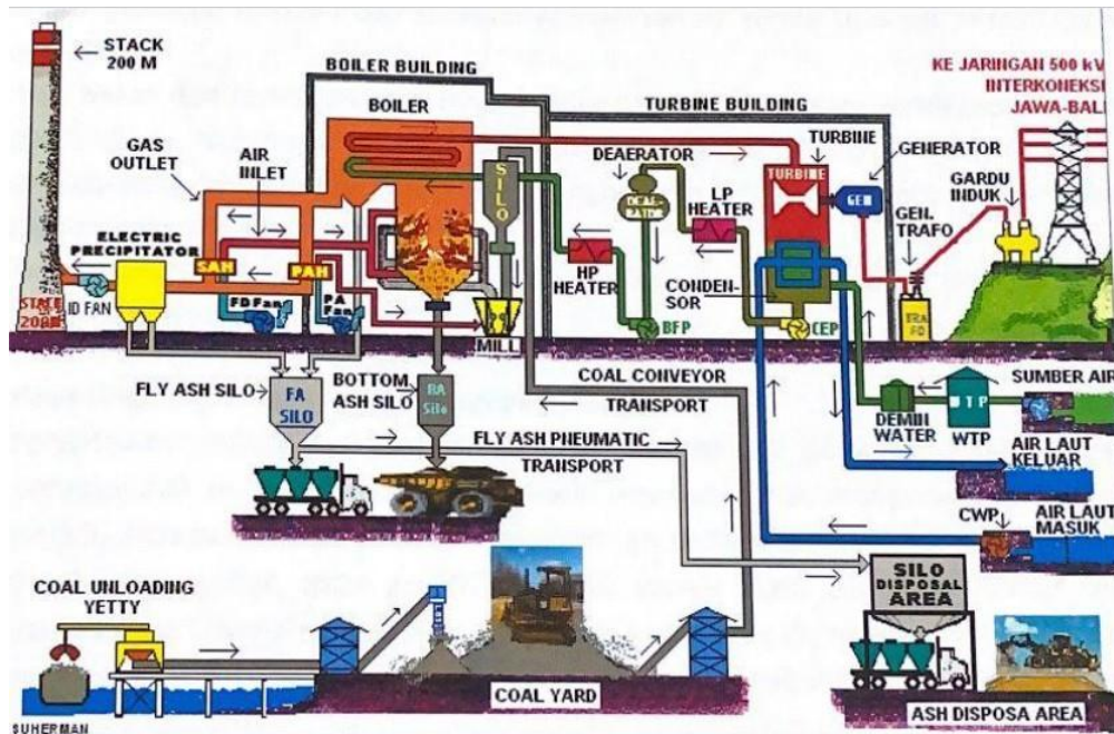
Gambar 3.2 Prinsip Kerja PLTU UP Paiton Unit 1 & 2
