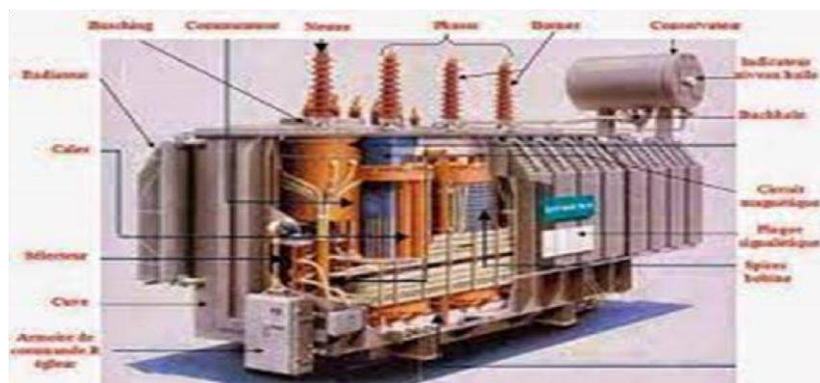
Gambar 2.37 Bagian Dalam Transformator
