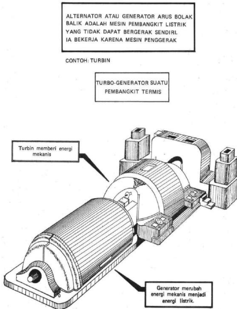
Gambar 2.36 Figure Generator bagian luar
