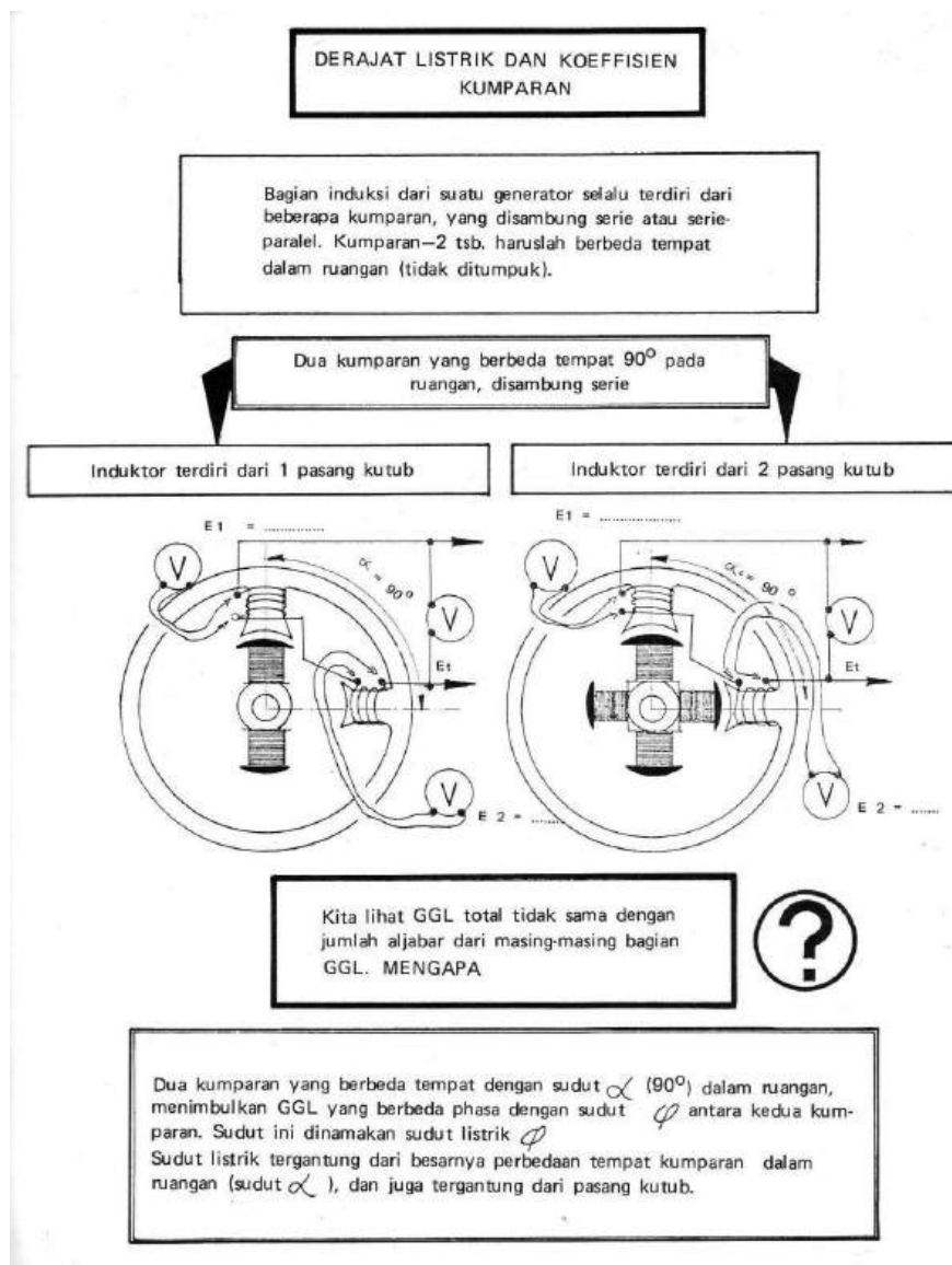
Gambar 2.35 Kumparan Bagian dalam Generator
