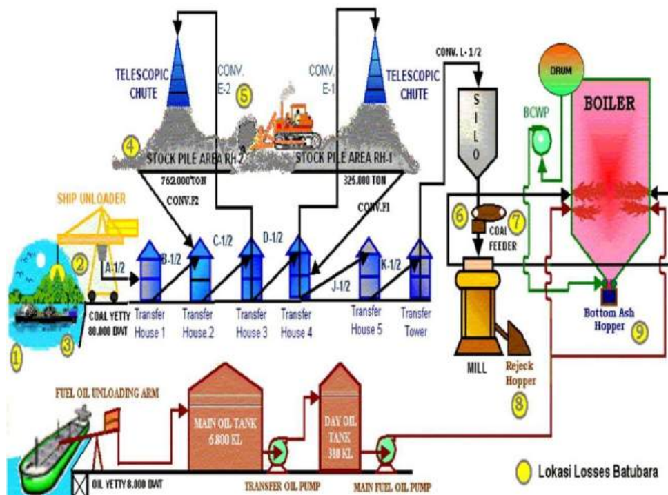
Gambar 2.17 Siklus Bahan Bakar PLTU
