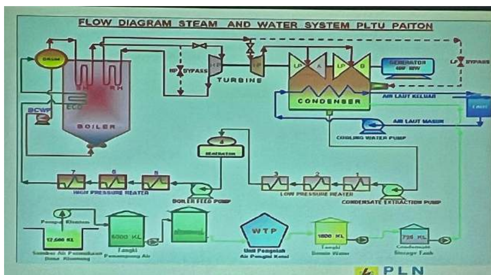
Gambar 2.15 Siklus Air Dan Uap
