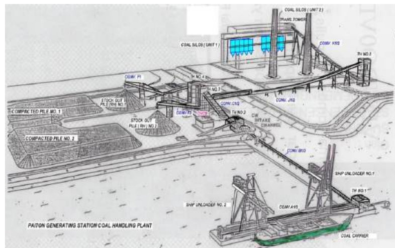
Gambar 2.19 Tempat Penimbunan Batu Bara
