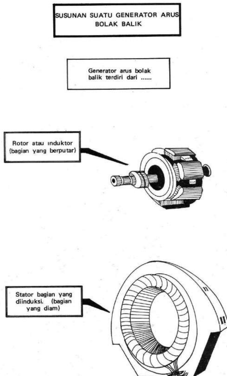
Gambar 2.34 Rotor dan Stator Generator
