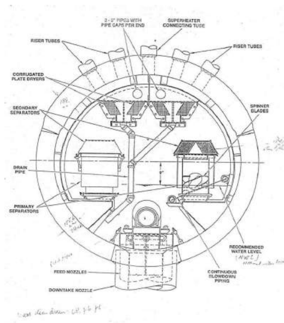
Gambar 2.28 Bagian dalam Steam Drum
