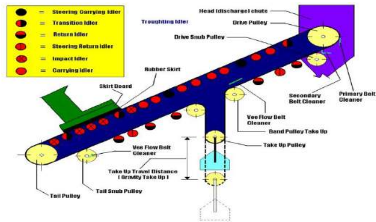
Gambar 2.20 System Conveyor pada Coal Handling
