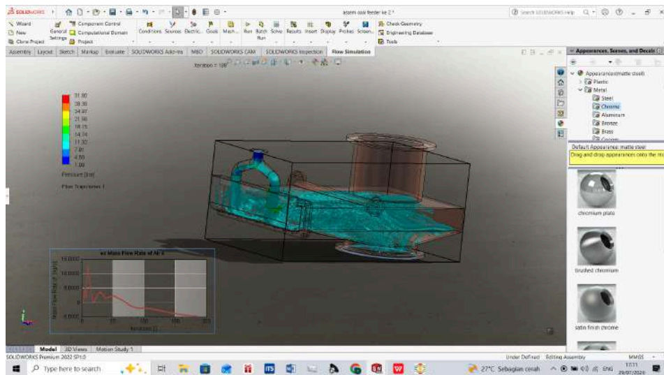
Gambar 5.5 Simulasi Aliran Udara Bertekanan
