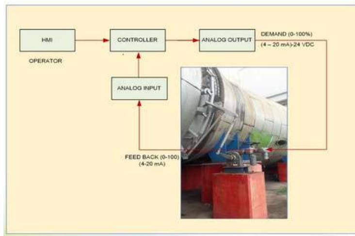
Gambar :5.5.6 Actuator motor Listrik untuk mengatur aliran di FD Fan
