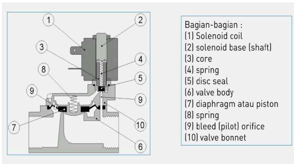
Gambar 5.5.9.Bagian-bagian Solenoide
