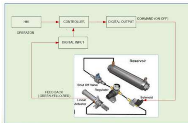
Gambar :5.5.5 .Rangkaian Solenoid dengan piston
