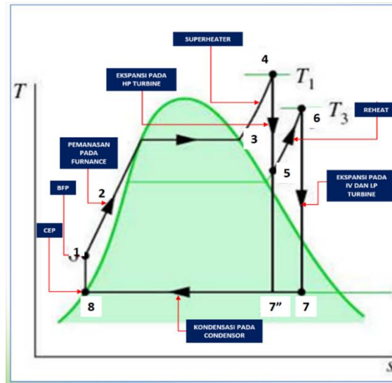
Gambar 3. 1 Konversi Energi dalam Siklus Rankine Di PLTU Paiton 9
