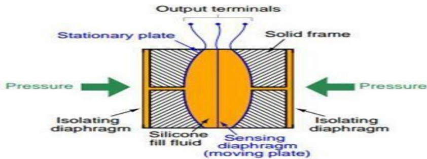
Gambar 3.2 Baaian – baaian dalam Diffrential Pressure Transmitter
