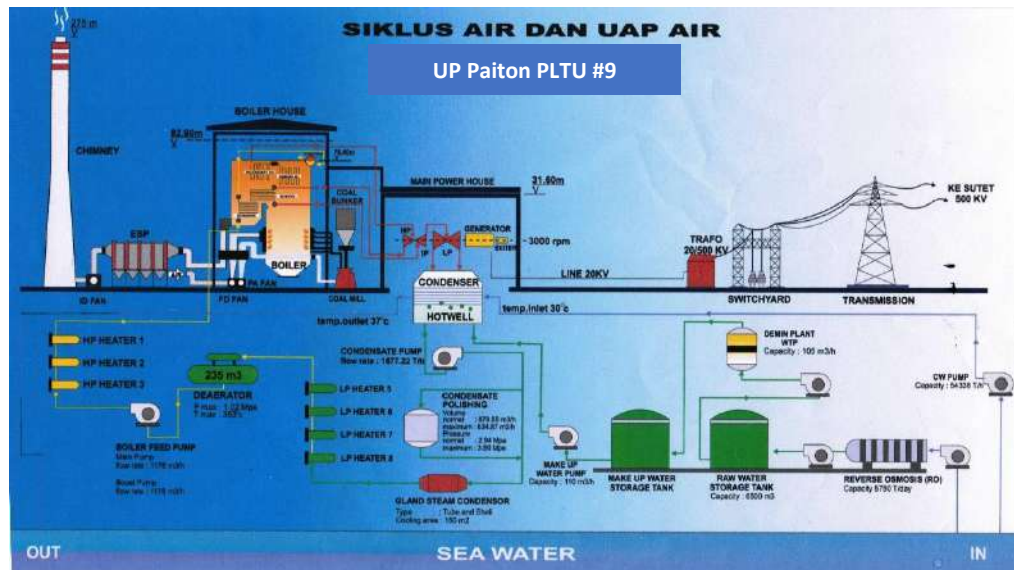
Gambar 2.1 Alur Proses PLTU Paiton 1,2, dan 9
