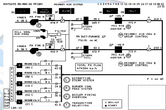
Gambar 0.13 Diagram Alur PA Fan
