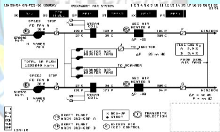
Gambar 0.12 Diagram Alur FD Fan
