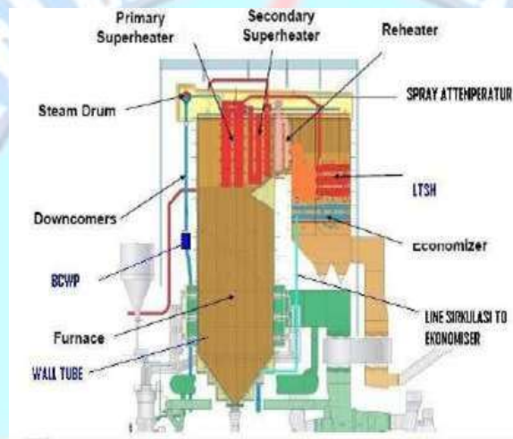
Gambar 0.21 Bagian Boiler
