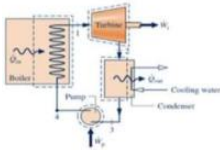
Gambar 3.2 Siklus Rankine Sumber : Moran et al., 2015
