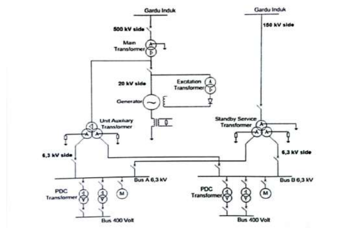
Gambar 2.10 Sistem Pola Operasi Kelistrikan PJB Unit 9 PLTU Paiton Baru (Sumber: Materi PT PLN NP UP Paiton)
