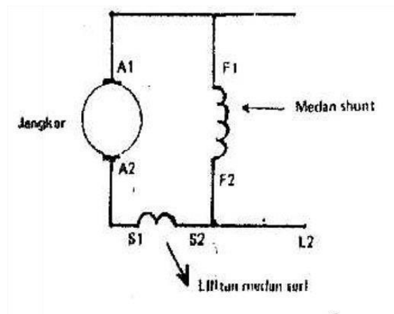
Gambar 2.26 Rangkaian Motor DC Kompon Panjang
