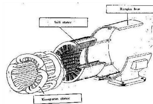
Gambar 2.16 Kontruksi Stator
