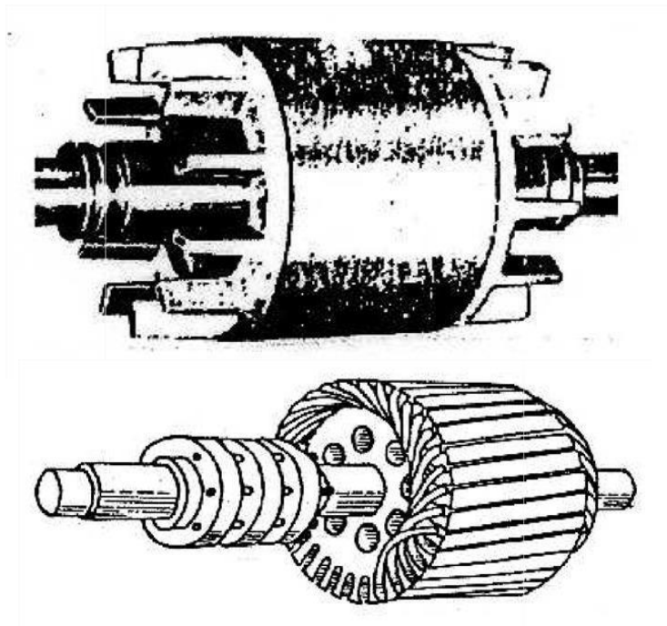
Gambar 2.17 Konstruksi Rotor Belitan
