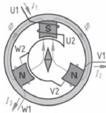
Gambar 2.19 Prinsip Kerja Motor Induksi 3 Phase
