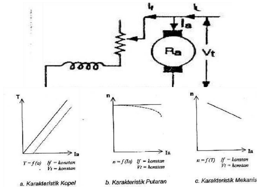
Gambar 2.24 Diagram dan Karakteristik Motor DC Shunt
