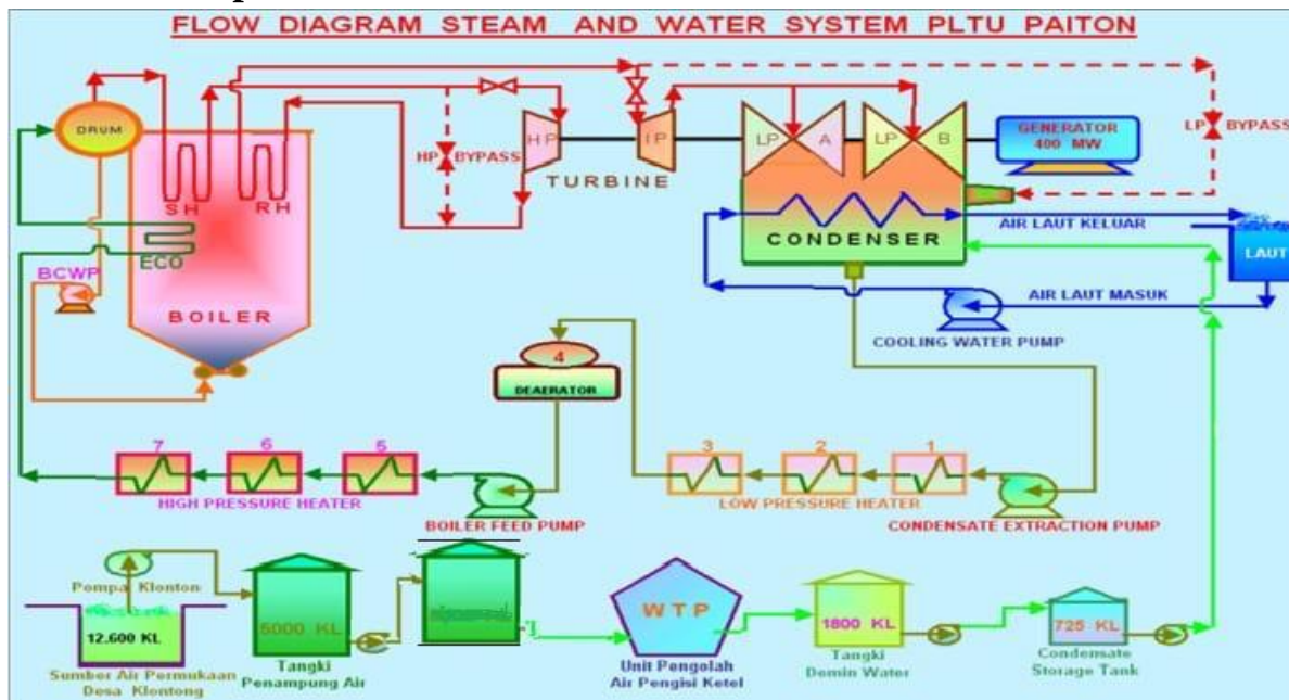
Gambar 2.11 Siklus Air dan Uap PLTU Paiton Unit 1&2
