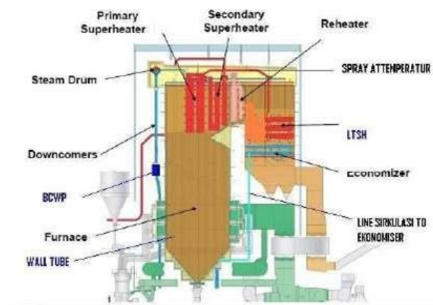
Gambar 2.12 Bagian Boiler
