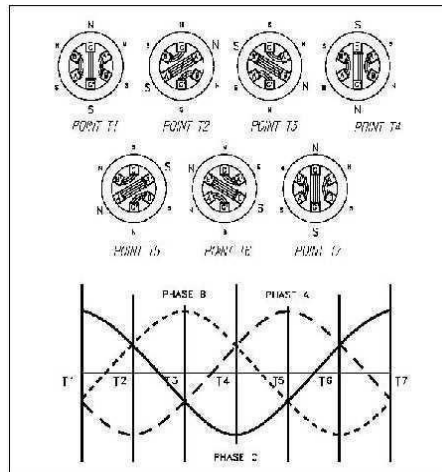
Gambar 2.18 Prinsip Kerja Motor Induksi
