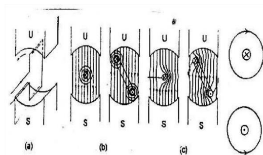
Gambar 2.22 Prinsip Kerja Motor Listrik Arus Searah
