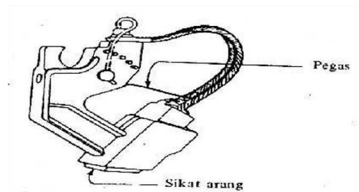
Gambar 2.21 Kontruksi Sikat Arang Motor DC
