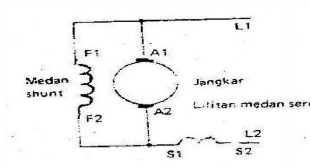
Gambar 2.25 Rangkaian Motor DC Kompon Pendek
