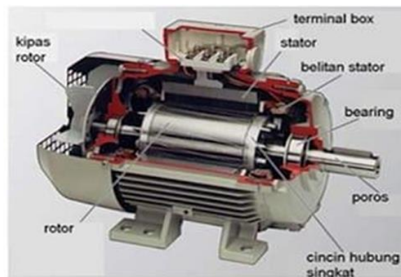
Gambar 2.15 Kontruksi Motor Listrik
