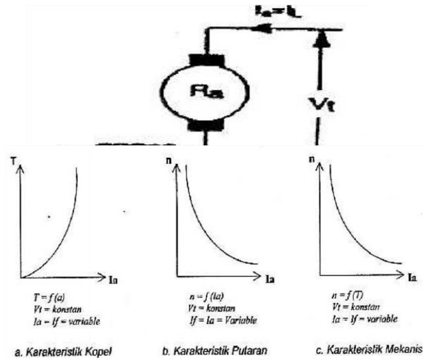
Gambar 2.23 Diagram Dan Karakteristik Motor DC Seri
