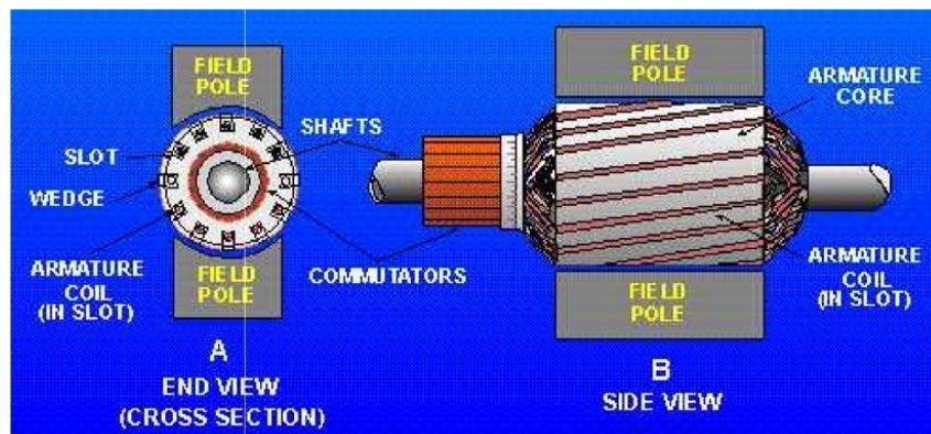
Gambar 2.20 Kontruksi Motor Listrik DC
