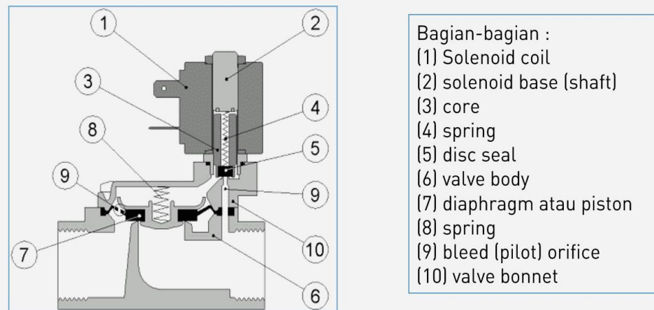
Gambar 5.5.9. Bagian-bagian Solenoide
