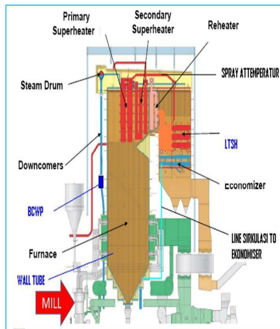
Gambar : 3.2 Boiler
