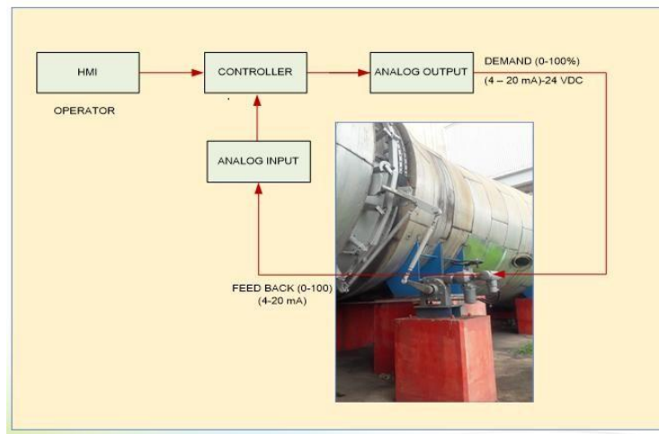
Gambar :5.5.6 Aktuator mator Listrik untuk mengatur aliran di FD Fan
