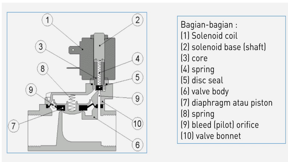
Gambar 5.5.9.Bagian-bagian Solenoide
