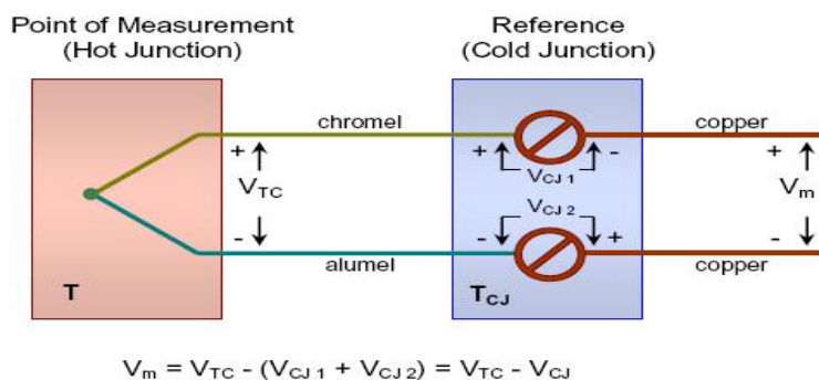
Gambar: 5.11 Rangkaian Thermocouple
