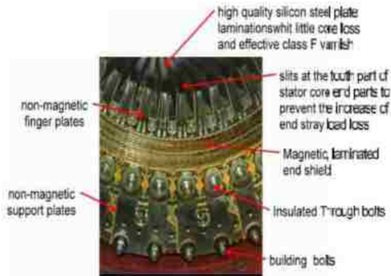
GAMBAR Rangkaian Stator di Generator.
