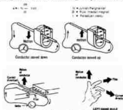
GAMBAR Rangkaian Generator.
