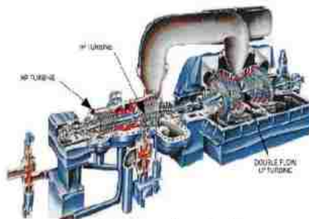
GAMBAR 30 Rangkaian Turbine
