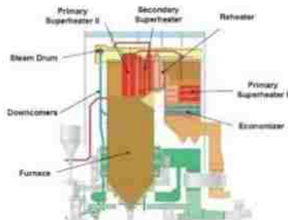
GAMBAR 9: Konstruksi Boiler Secara Sederhana
