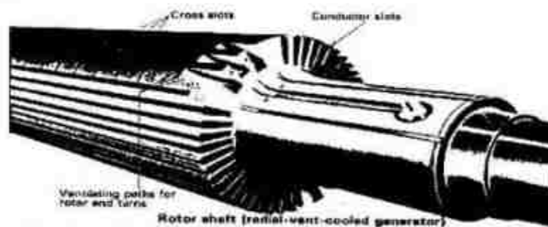
GAMBAR Rangkaian Rotor
