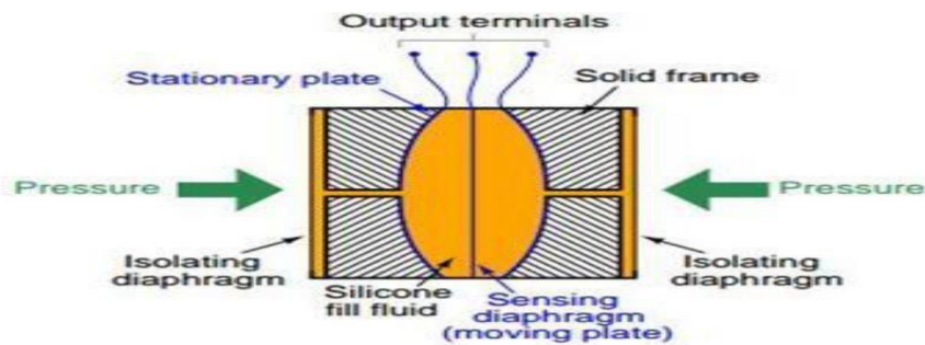
Gambar 3.2 Bagian – bagian dalam Diffrential Pressure Transmitter
