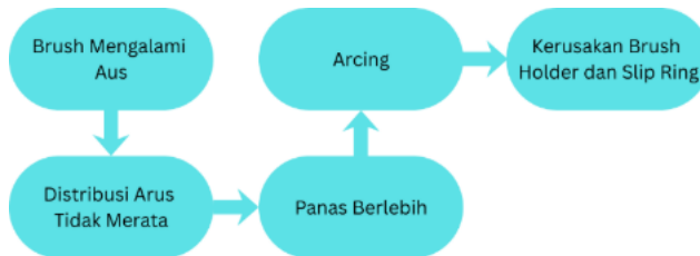
Gambar IV.13 Diagram alir kerusakan brush
