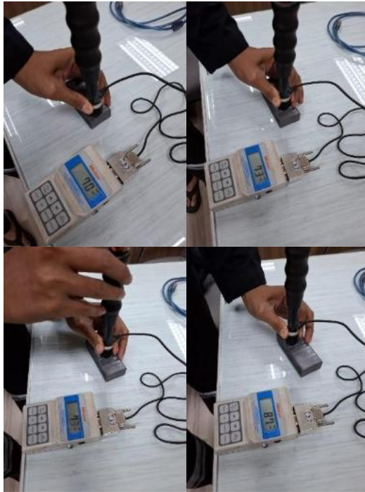
Gambar IV.10 Pengujian kekerasan brush baru
