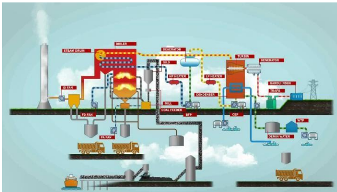
Gambar III.1 Diagram alir PLTU Paiton unit 1 dan 2
