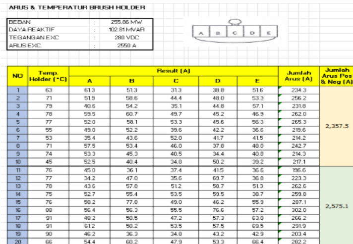
Gambar IV.11 Data pengukuran arus dan temperature brush setelah dilakukan penggantian.
