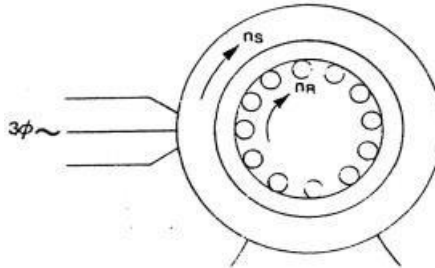
Gambar III.9 Prinsip kerja motor induksi
