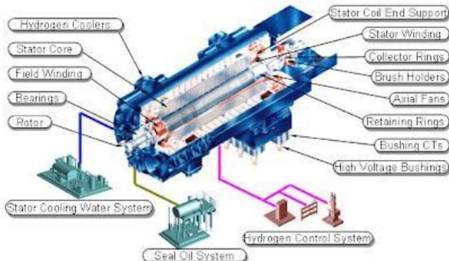
Gambar IV.1 Struktur Generator
