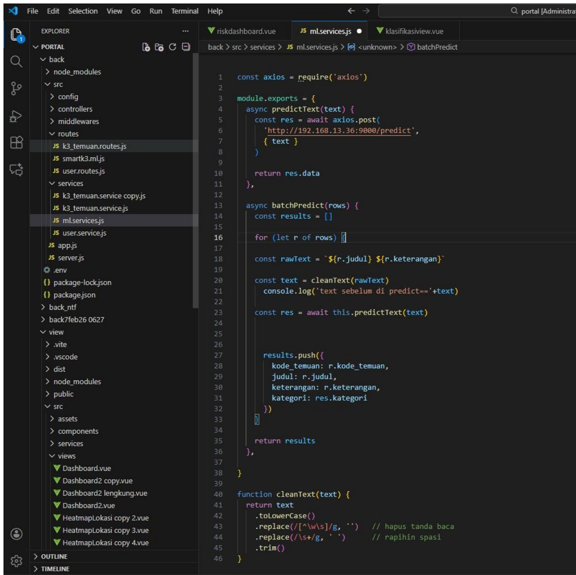
Gambar 4.7.5 Implementasi Integrasi Layanan Prediksi IndoBERT pada Backend Web K3
