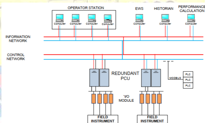
Gambar5. 2.1Komponen DCS
