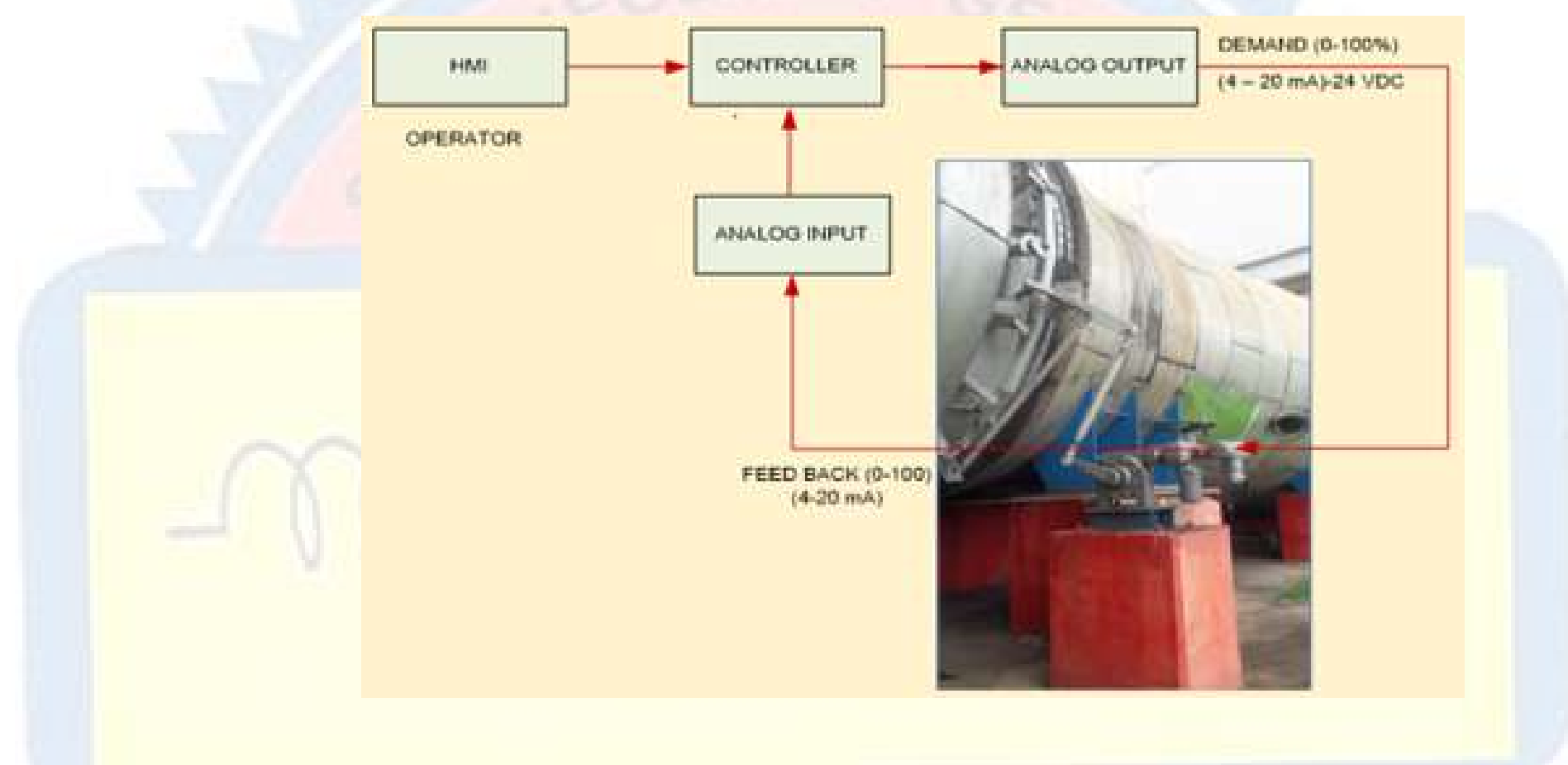
Gambar5. 16 Actuator Motor Listrik untuk mengatur aliran di FD Fan
