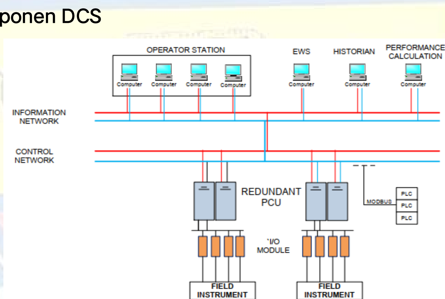
Gambar5. 2.1Komponen DCS
