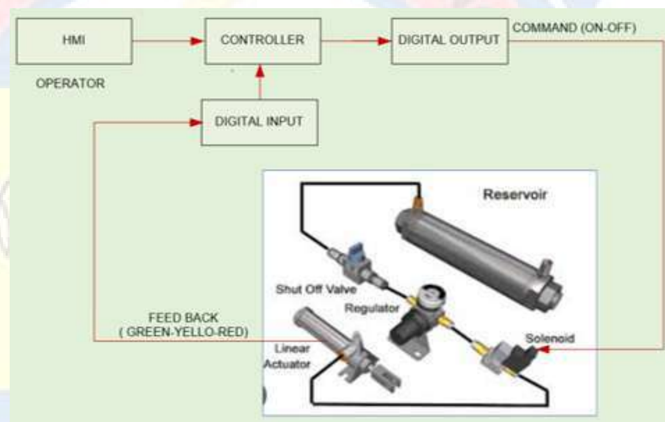
Gambar5. 15 Rangkaian Solenoide dengan Piston
