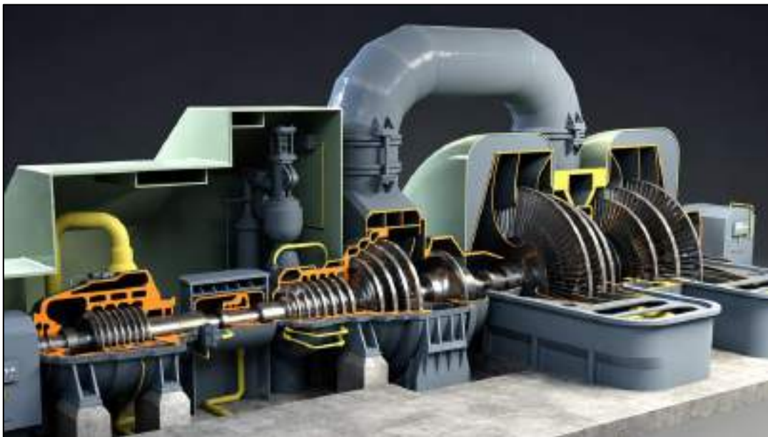
Gambar 3. 4 Potongan Melintang Susunan Konstruksi Turbin Uap Tipe HP, IP, dan LP
