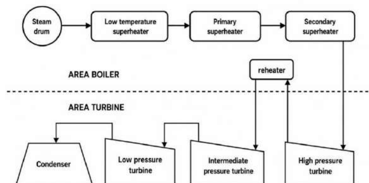
Gambar 3.8 Siklus Uap
