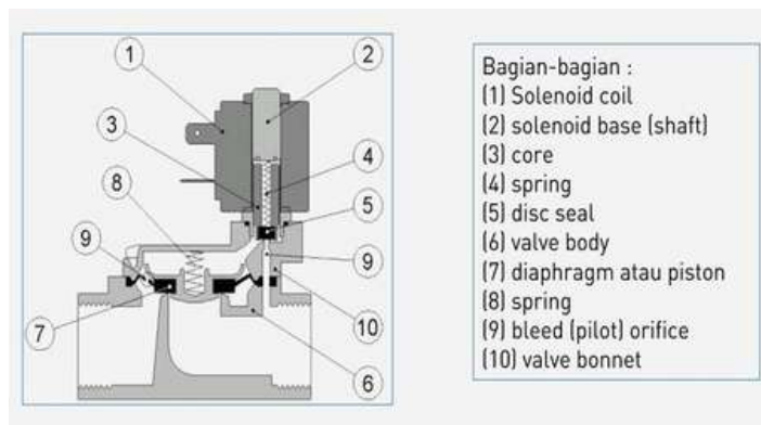
Gambar 5.18 Bagian-bagian Solenoide
