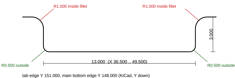
DETAIL J3_TAB (scale 6.0 : 1)
