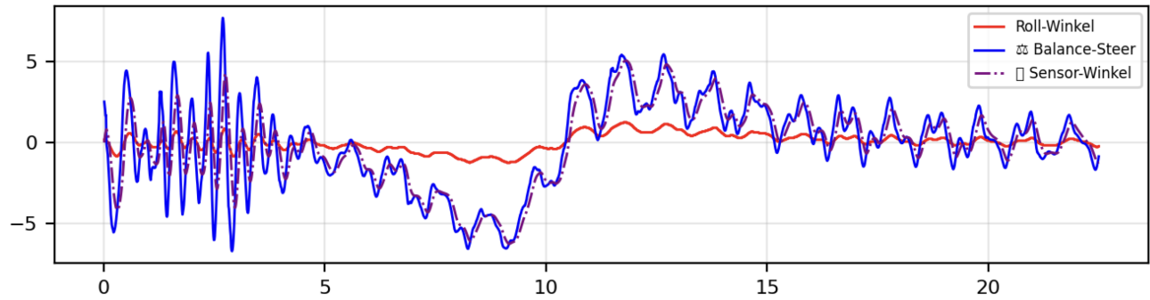
Abbildung 48: Zeitverläufe mit angepasstem Balance PID (Fall E, M = 4,0\text{ m} ).
