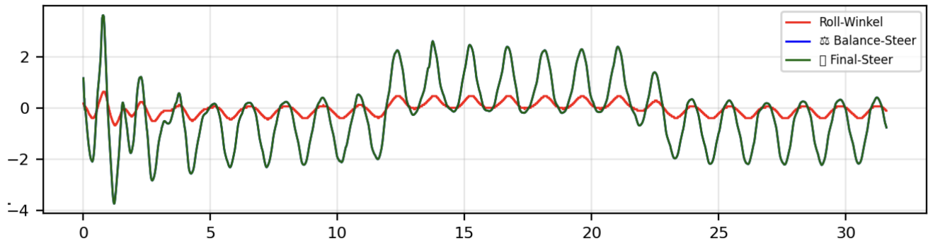
Abbildung 37: Zeitreihen bei 1,0 m/s mit erhöhten Gains: gedämpfter Rollwinkelverlauf; höhere, aber tolerierbare Lenkaktivität (keine Sättigung, keine Divergenz).
