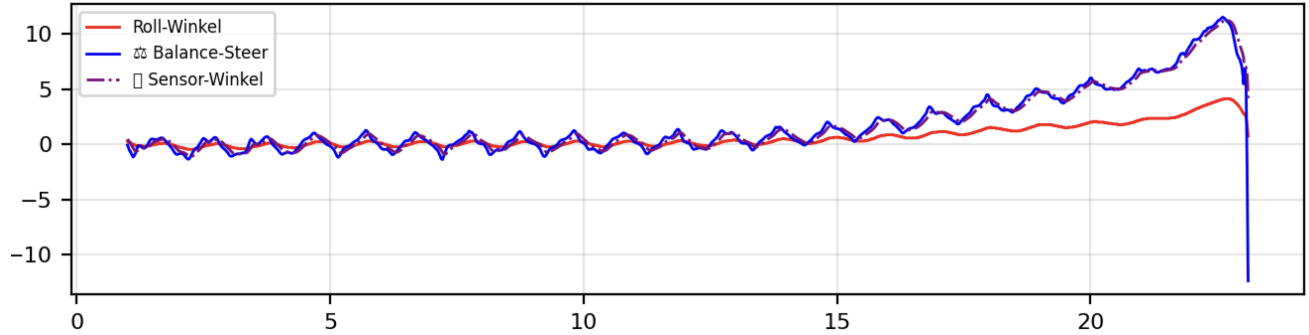
Abbildung 42: Zeitverläufe Rollwinkel/Balancelenkung (Fall B, M = 2,0 m, Baseline-Gewichte).
