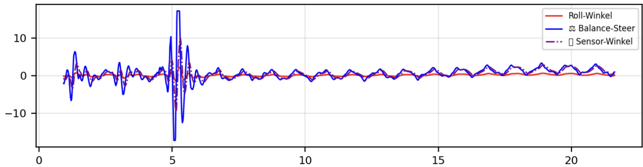
Abbildung 44: Zeitverläufe mit retuntem Balance-PID (Fall B, M = 2,0 m).
