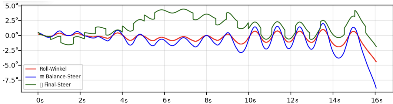
Abbildung 14: Kurvenfahrt mit reinem P-Regler (Zeitreihen)
