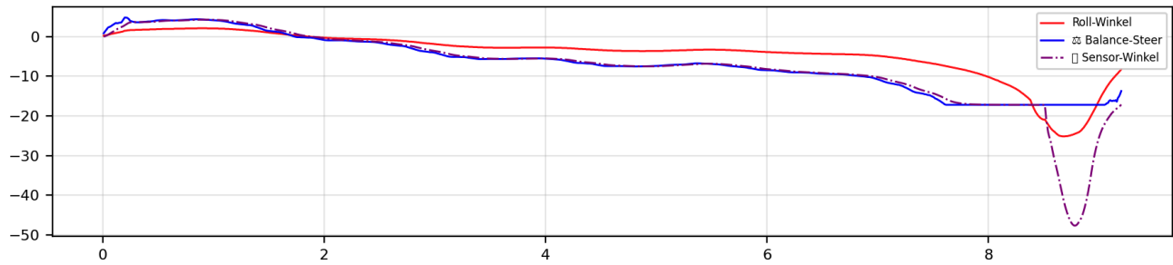
Abbildung 35: Zeitverlauf bei 1,0 m/s (Baseline-Regler): ansteigende Rollauslenkung und instabiles Verhalten nach \approx 7 s.
