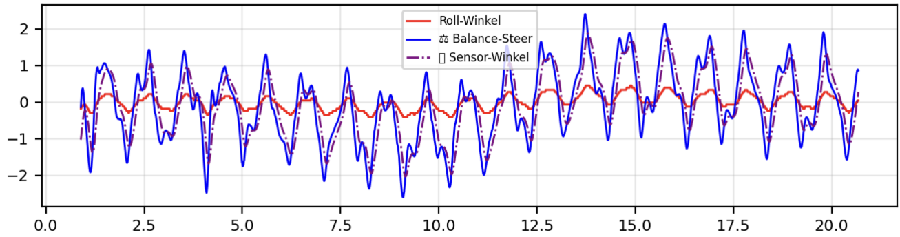
Abbildung 46: Zeitverläufe mit angepasstem Balance PID (Fall D, M = 2,0 \text{ m} ).
