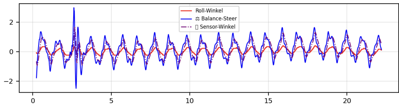
Abbildung 40: Zeitverläufe Rollwinkel/Balancelenkung (Fall A, M = 1,0 m).
