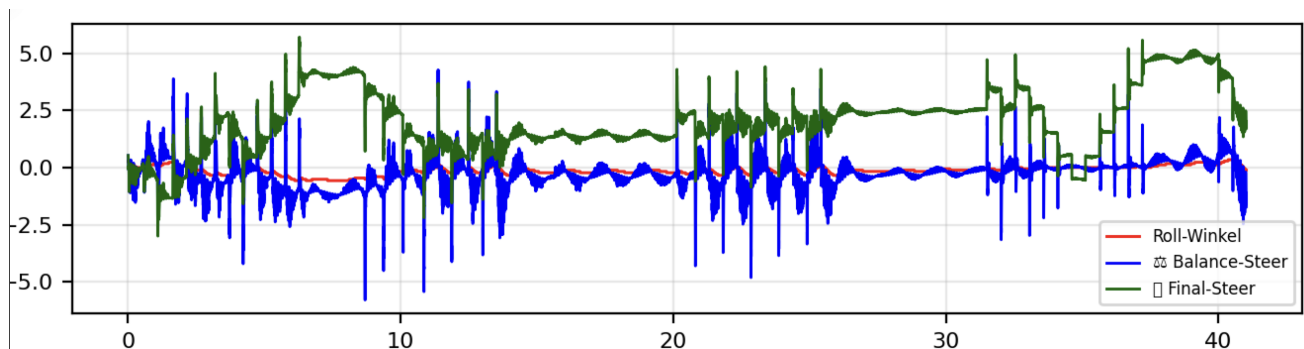
Abbildung 21: Kurvenfahrt mit PID-Regler und ROI-Fallback-Erkennung
