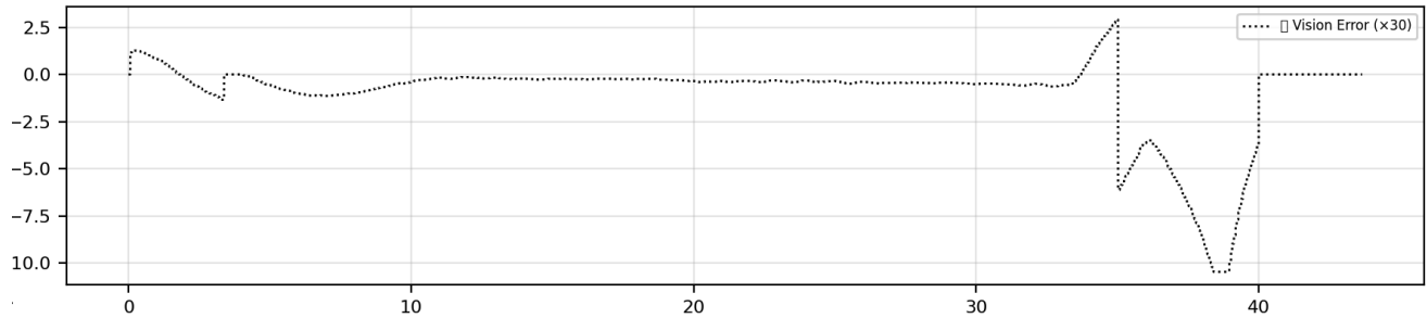
Abbildung 22: ROI-Querfehler während der PID-Regler-Fahrt (ROI)
