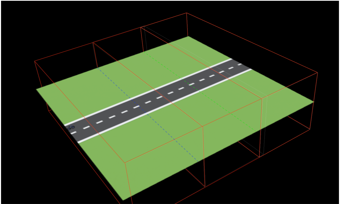
Abbildung 31: Versuchsaufbau: Gerade Strecke mit drei seitlichen Windkanälen (rote Drahtgitterboxen). Die Fahrbahnmittte dient als Referenz für die Spurführung.
