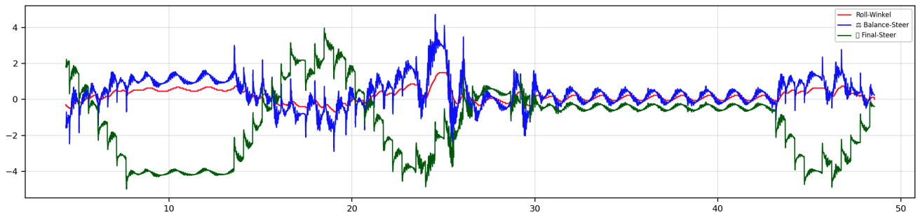
Abbildung 26: S-Kurve: ausgewählte Zeitreihen (Rollwinkel, Balance-Soll, final_steer )
