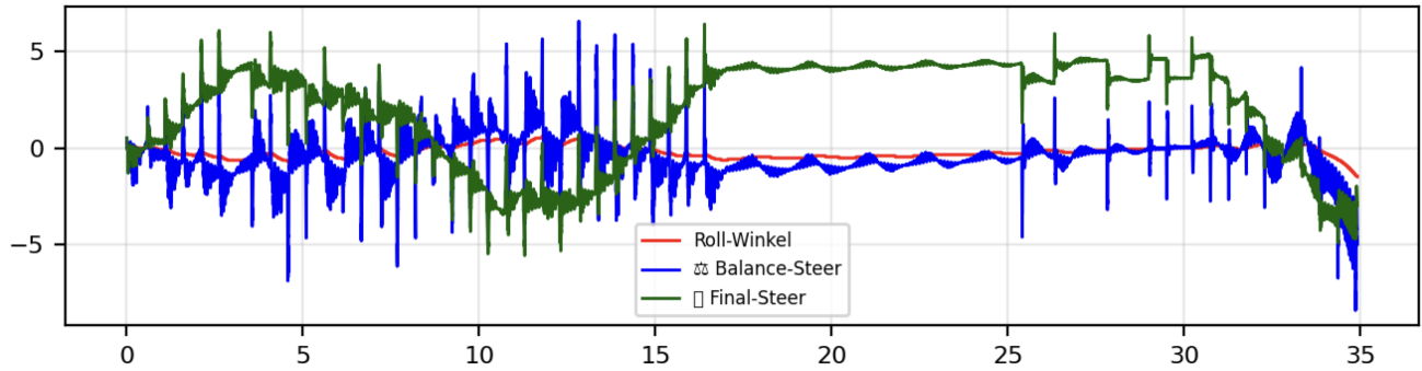
Abbildung 17: Kurvenfahrt mit PID-Regler und YOLO-Spurführung
