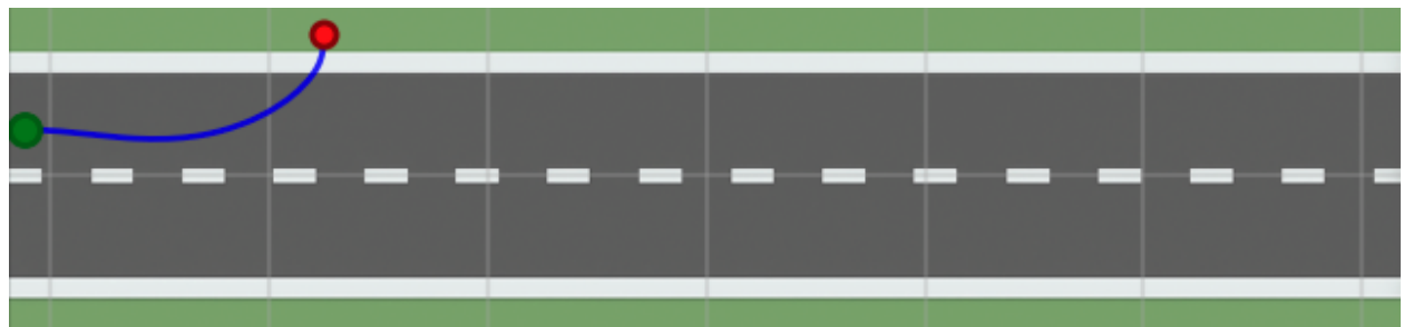
Figure 34: Trajektorie bei 1,0 m/s Seitenwind (Baseline-Gains): starke Abdrift nach rechts mit vorzeitigem Abbruch infolge Umkippens.
