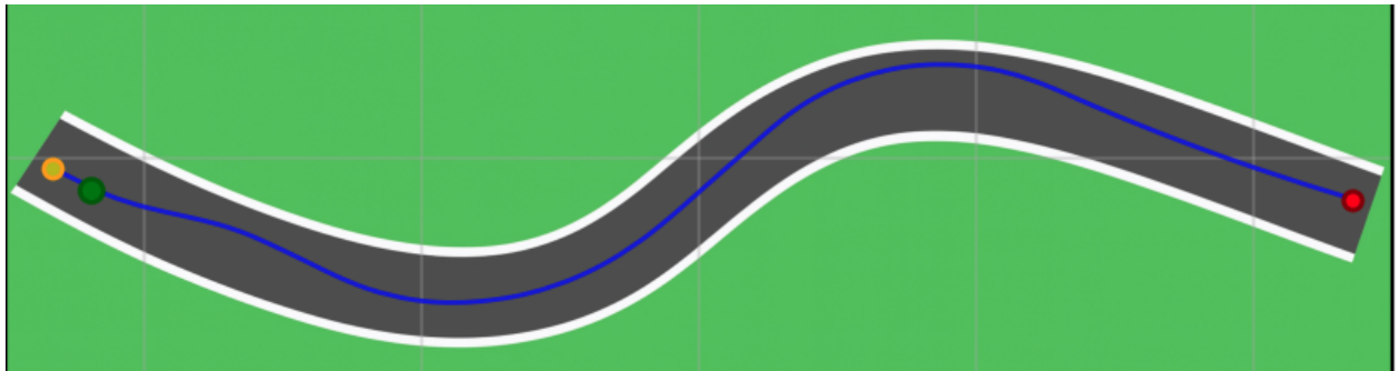
Figure 28: S-Kurve mit ROI-Regler
