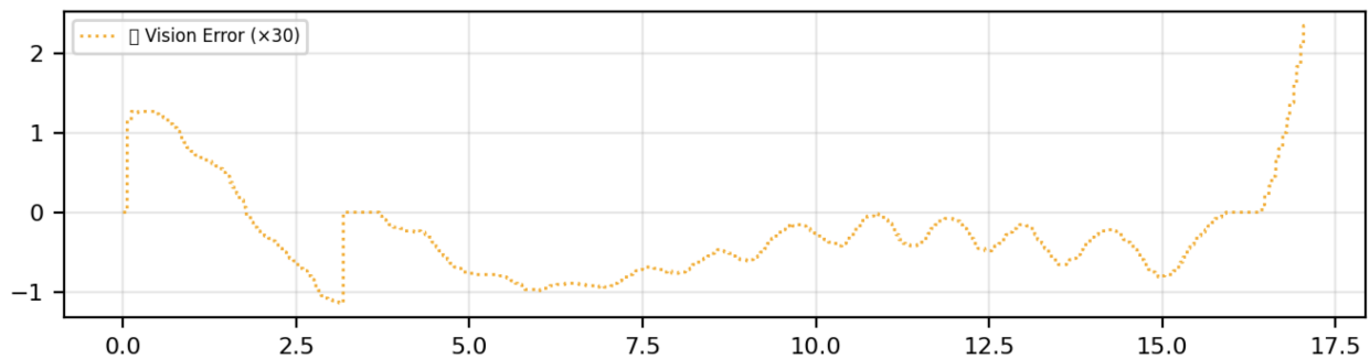
Figure 15: ROI-Querfehler während der P-Regler-Fahrt
