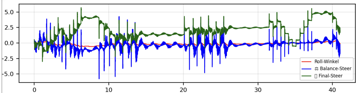
Figure 21: Kurvenfahrt mit PID-Regler und ROI-Fallback-Erkennung
