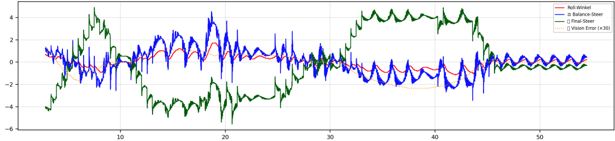
Figure 29: S-Kurve mit ROI-Regler Daten
