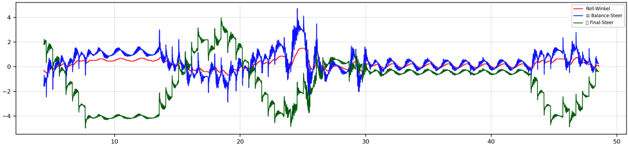
Figure 26: S-Kurve: ausgewählte Zeitreihen (Rollwinkel, Balance-Soll, final_steer )
