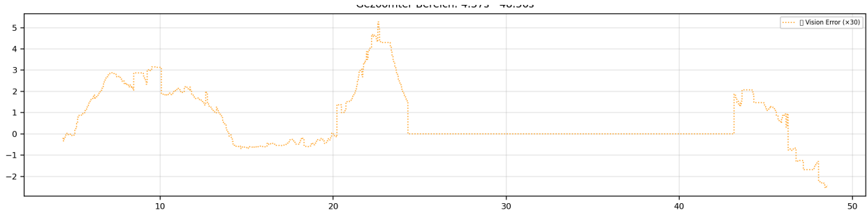
Figure 27: S-Kurve: visionbasierter Querfehler \tilde{e}_y
