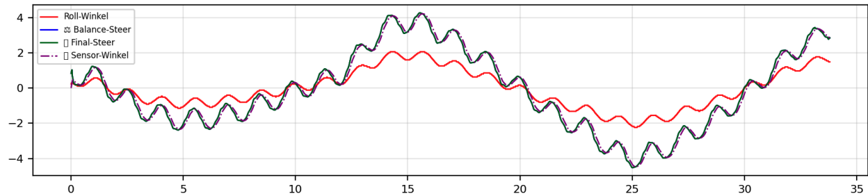
Figure 33: Zeitreihen bei 0,5 m/s Seitenwind: Rollwinkel, Balance-Steer und finales Lenkkommando. Die Richtung der Seitenböe spiegelt sich in der Vorzeichenfolge des Rollwinkels wider; der D-Anteil dämpft die schnelle Nick-/Roll-Dynamik.
