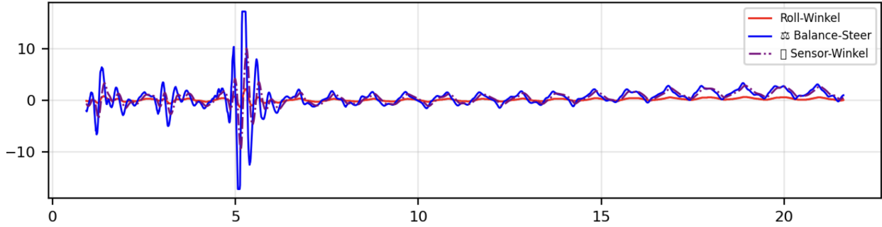
Figure 44: Zeitverläufe mit retuntem Balance-PID (Fall B, M = 2,0 m).
