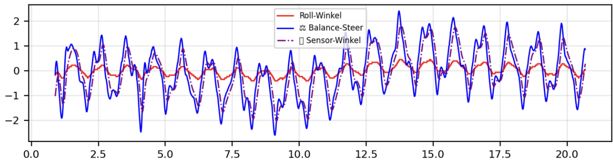
Figure 46: Zeitverläufe mit angepasstem Balance PID (Fall D, M = 2,0 m).
