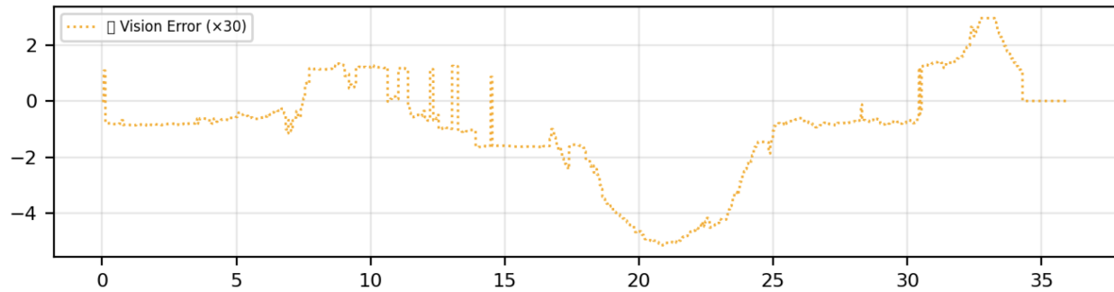
Figure 18: ROI-Querfehler während der PID-Regler-Fahrt (YOLO)
