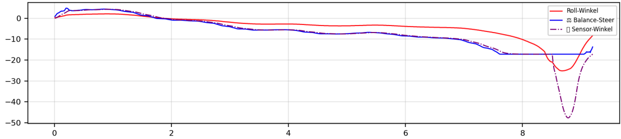
Figure 35: Zeitverlauf bei 1,0 m/s (Baseline-Gains): ansteigende Rollauslenkung und instabiles Verhalten nach \approx 7 s.
