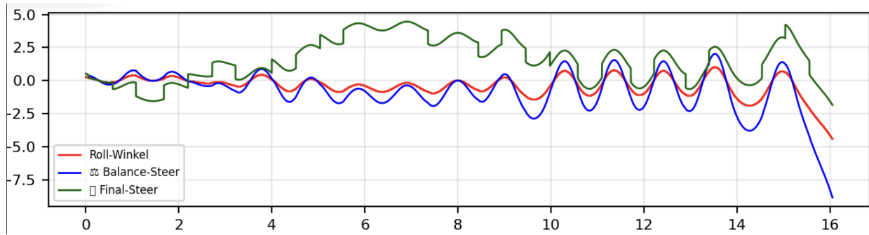
Figure 14: Kurvenfahrt mit reinem P-Regler (Zeitreihen)
