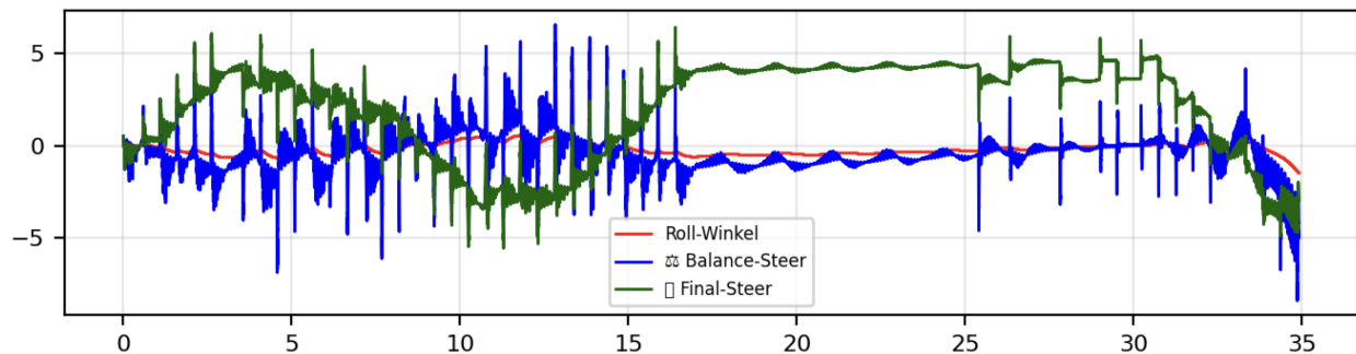
Figure 17: Kurvenfahrt mit PID-Regler und YOLO-Spurführung
