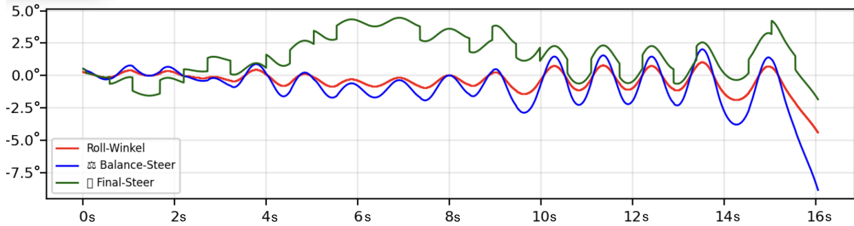
Abbildung 14: Kurvenfahrt mit reinem P-Regler (Zeitreihen). X-Achse: Zeit in Sekunden, Y-Achse: Winkel in Grad
