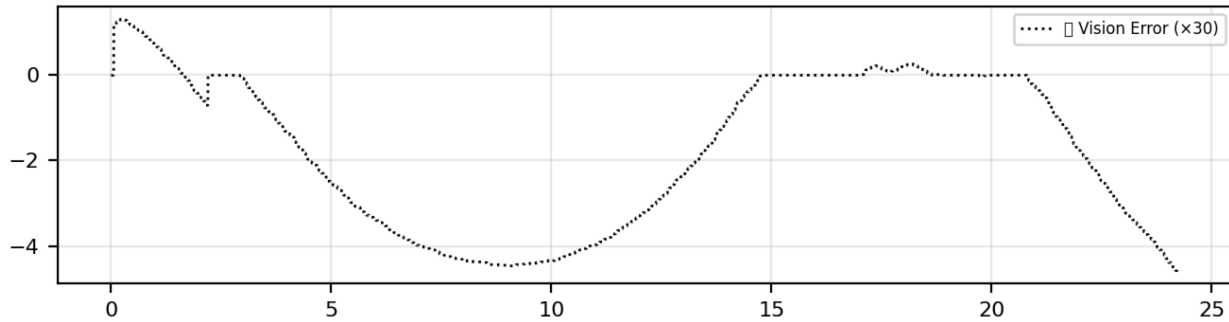
Abbildung 25: ROI-Querfehler während der P-Regler-Fahrt (Vision)
