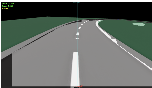
(a) Korrekte Fahrbahnsegmentierung
