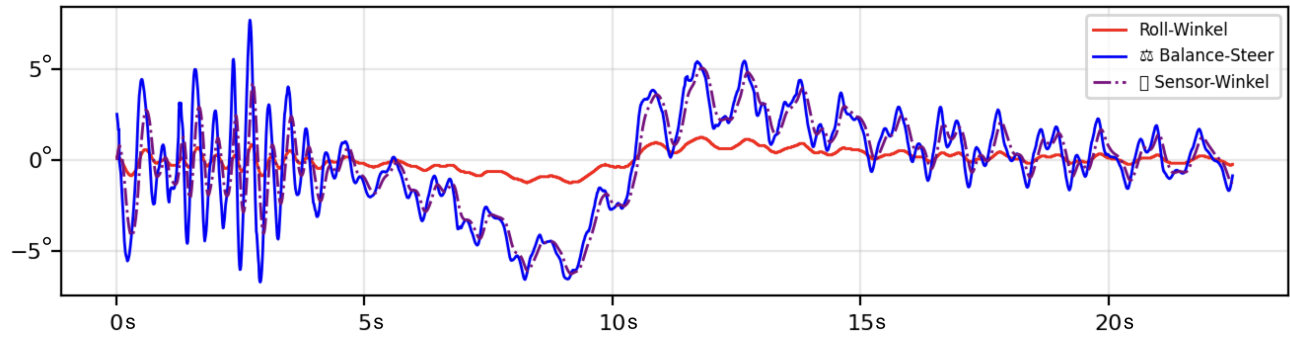
Abbildung 48: Zeitverläufe mit angepasstem Balance PID (Fall E, M = 4,0 m). X-Achse: Zeit in Sekunden, Y-Achse: Winkel in Grad
