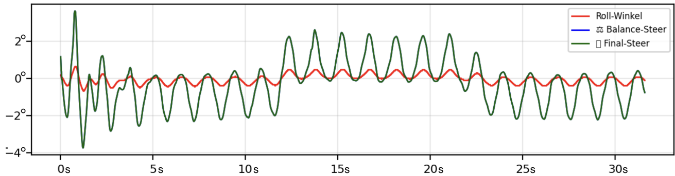
Abbildung 37: Zeitreihen bei 1,0 m/s mit erhöhten Gains: gedämpfter Rollwinkelverlauf; höhere, aber tolerierbare Lenkaktivität (keine Sättigung, keine Divergenz). X-Achse: Zeit in Sekunden, Y-Achse: Winkel in Grad
