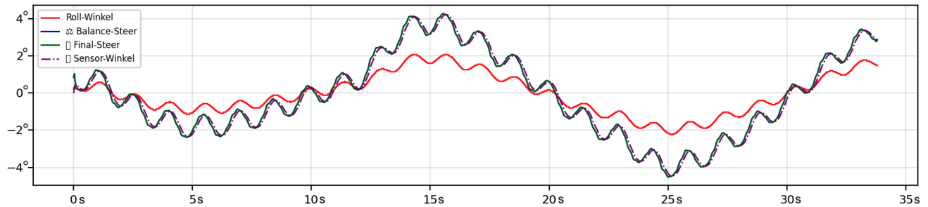
Abbildung 33: Zeitreihen bei 0,5 m/s Seitenwind: Rollwinkel, Balance-Steer und finales Lenkkommando. Die Richtung der Seitenböe spiegelt sich in der Vorzeichenfolge des Rollwinkels wider; der D-Anteil dämpft die schnelle Nick-/Roll-Dynamik. X-Achse: Zeit in Sekunden, Y-Achse: Winkel in Grad
