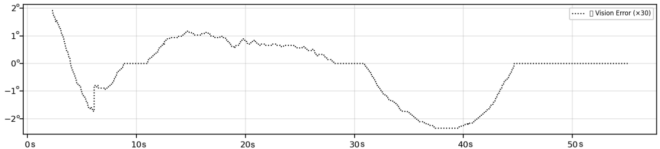
Abbildung 30: S-Kurve mit ROI-Regler Error
