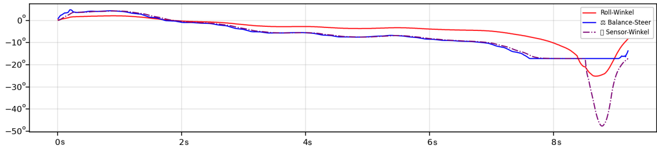
Abbildung 35: Zeitverlauf bei 1,0 m/s (Baseline-Regler): ansteigende Rollauslenkung und instabiles Verhalten nach \approx 7 s. X-Achse: Zeit in Sekunden, Y-Achse: Winkel in Grad
