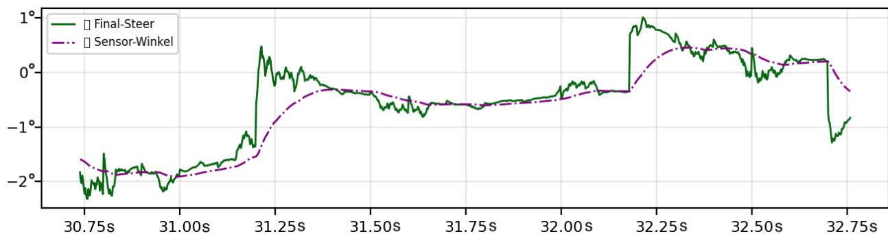
Abbildung 6: Lenk-Sollwert und Lenk-Istwert.
