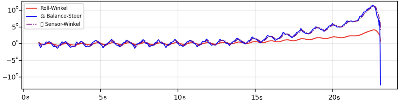
Abbildung 42: Zeitverläufe Rollwinkel/Balancelenkung (Fall B, M = 2,0 m, Baseline-Gewichte). X-Achse: Zeit in Sekunden, Y-Achse: Winkel in Grad
