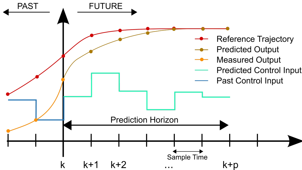
Abbildung 1: Verständnisschema der MPC-Regelung
