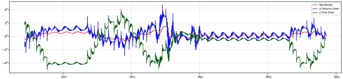
Abbildung 26: S-Kurve: ausgewählte Zeitreihen (Rollwinkel, Balance-Soll, final_steer ). X-Achse: Zeit in Sekunden, Y-Achse: Winkel in Grad
