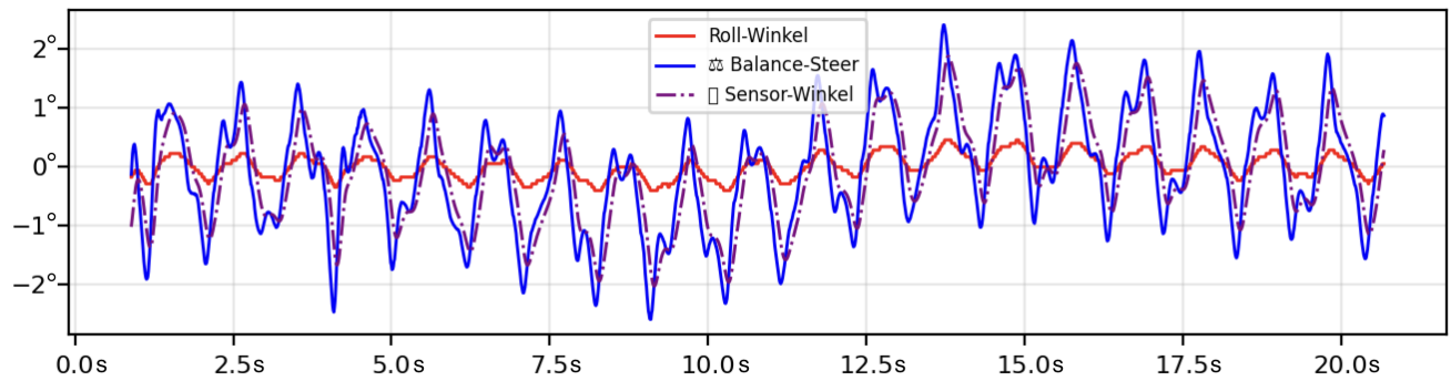
Abbildung 46: Zeitverläufe mit angepasstem Balance PID (Fall D, M = 2,0\text{m} ). X-Achse: Zeit in Sekunden, Y-Achse: Winkel in Grad
