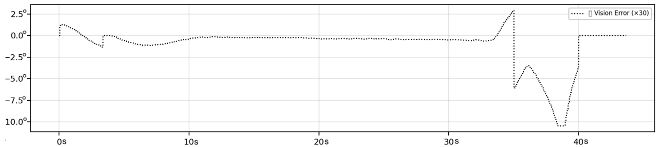
Abbildung 22: ROI-Querfehler während der PID-Regler-Fahrt (ROI)
