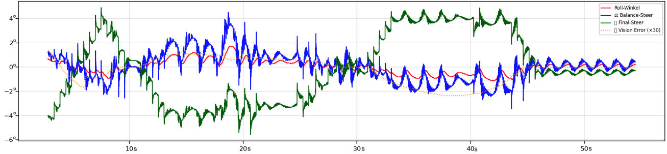
Abbildung 29: S-Kurve mit ROI-Regler Daten. X-Achse: Zeit in Sekunden, Y-Achse: Winkel in Grad
