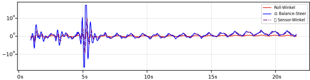
Abbildung 44: Zeitverläufe mit retuntem Balance-PID (Fall B, M = 2,0 m). X-Achse: Zeit in Sekunden, Y-Achse: Winkel in Grad
