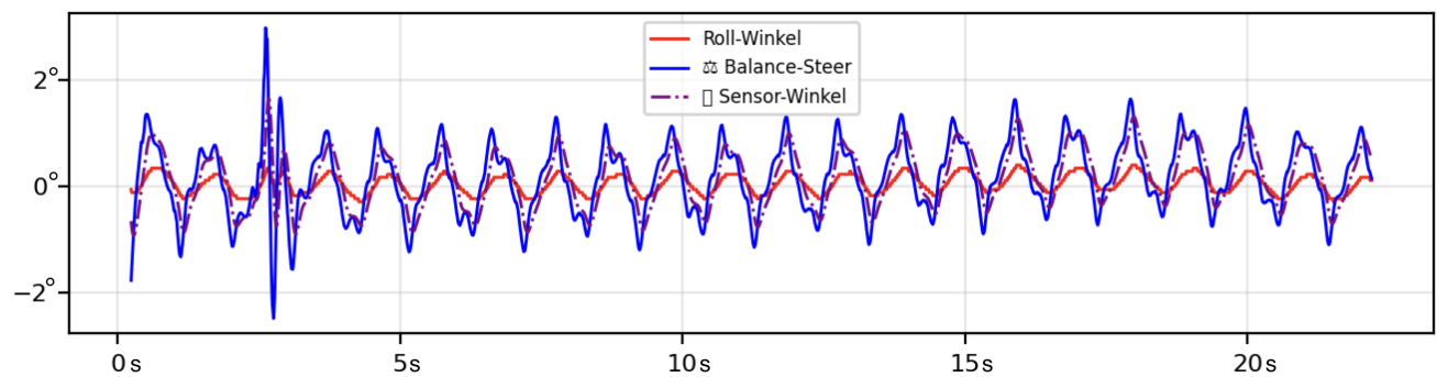
Abbildung 40: Zeitverläufe Rollwinkel/Balancelenkung (Fall A, M = 1,0 m). X-Achse: Zeit in Sekunden, Y-Achse: Winkel in Grad
