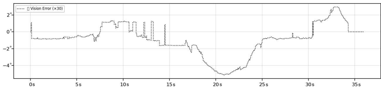
Abbildung 18: ROI-Querfehler während der PID-Regler-Fahrt (YOLO)
