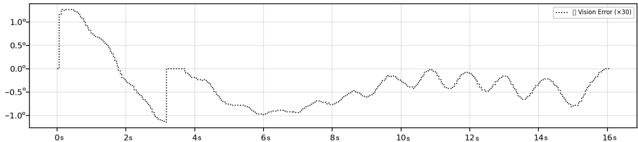
Abbildung 15: ROI-Querfehler während der P-Regler-Fahrt
