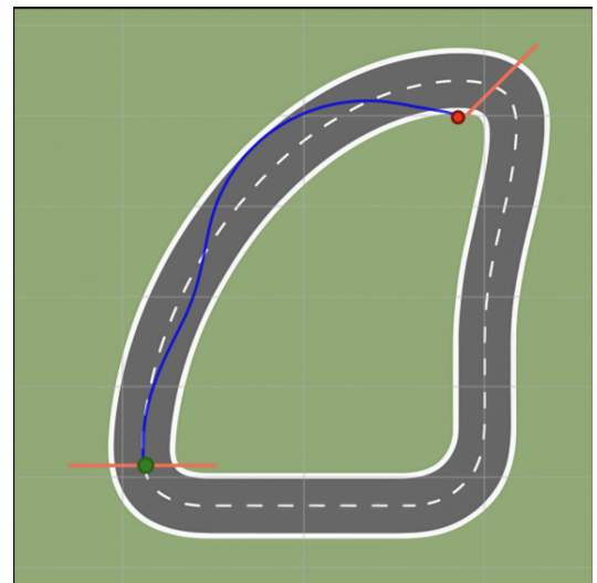
Abbildung 19: Gefahrene Trajektorie (PID-Regler mit YOLO)
