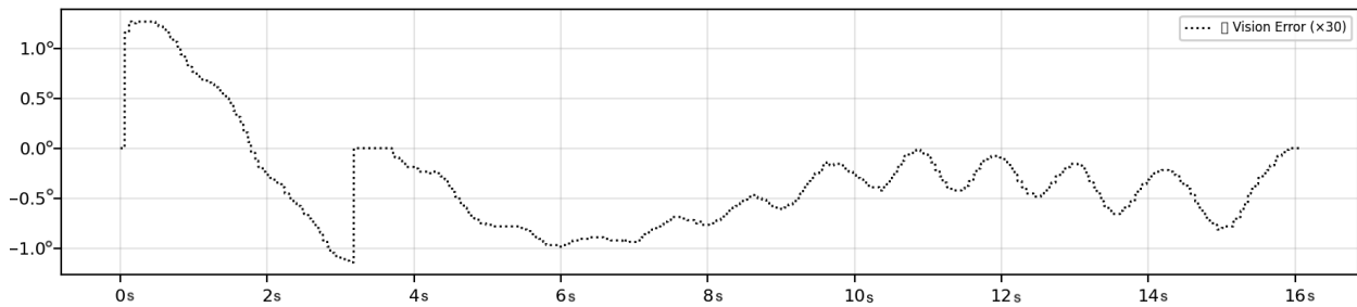
Abbildung 15: ROI-Querfehler während der P-Regler-Fahrt
