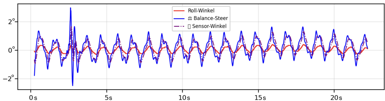
Abbildung 43: Zeitverläufe Rollwinkel/Balancelenkung (Fall A, M = 1,0 m). X-Achse: Zeit in Sekunden, Y-Achse: Winkel in Grad
