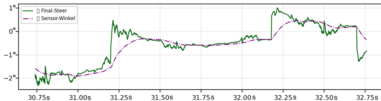
Abbildung 6: Lenk-Sollwert und Lenk-Istwert.
