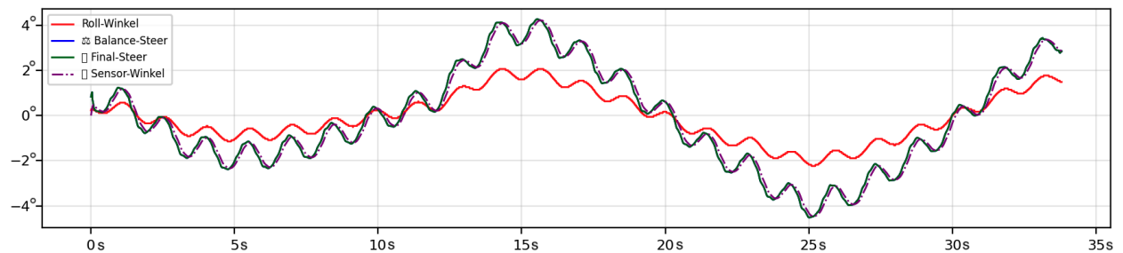
Abbildung 36: Zeitreihen bei 0,5 m/s Seitenwind: Rollwinkel, Balance-Steer und finales Lenkkommando. Die Richtung der Seitenböe spiegelt sich in der Vorzeichenfolge des Rollwinkels wider; der D-Anteil dämpft die schnelle Nick-/Roll-Dynamik. X-Achse: Zeit in Sekunden, Y-Achse: Winkel in Grad
