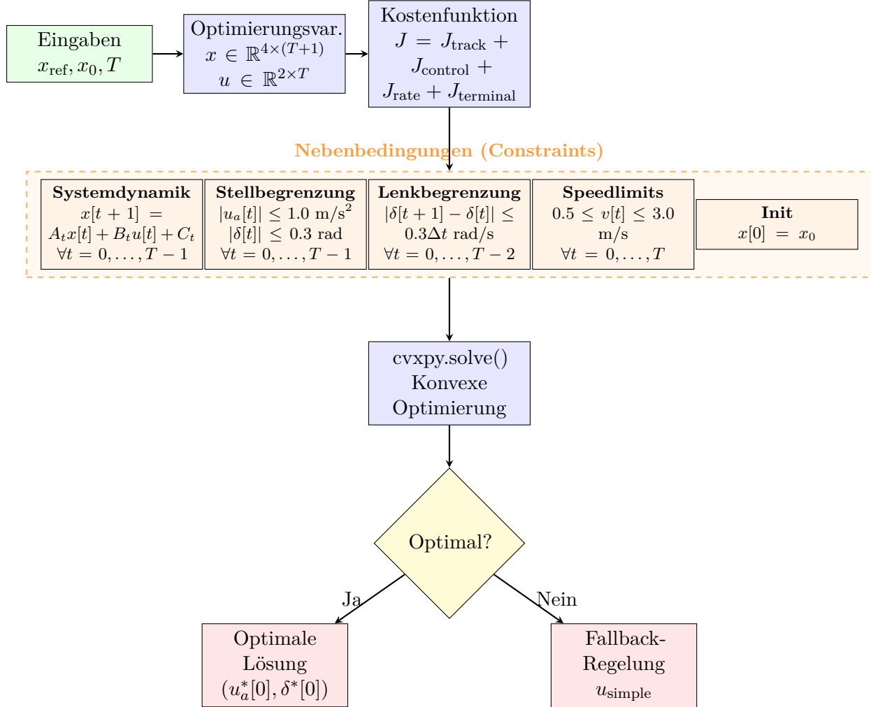
Abbildung 9: MPC-Optimierungsalgorithmus mit gebündelten Nebenbedingungen
