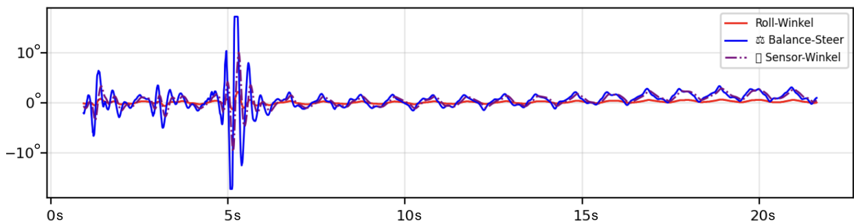
Abbildung 47: Zeitverläufe mit retuntem Balance-PID (Fall B, M = 2,0 m). X-Achse: Zeit in Sekunden, Y-Achse: Winkel in Grad
