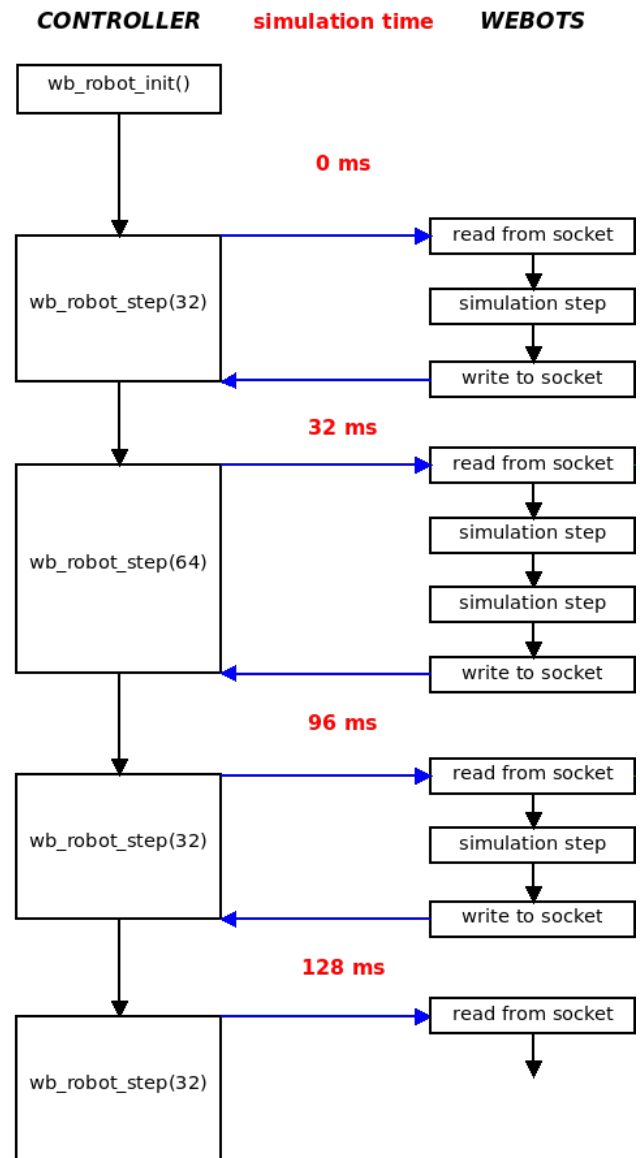
Abbildung 8: Synchronisation zwischen Controller und Simulation.
