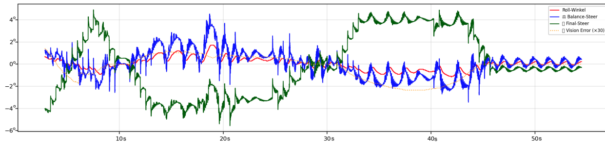
Abbildung 32: S-Kurve mit ROI-Regler Daten. X-Achse: Zeit in Sekunden, Y-Achse: Winkel in Grad
