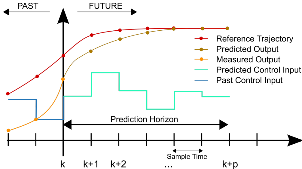
Abbildung 1: Verständnisschema der MPC-Regelung
