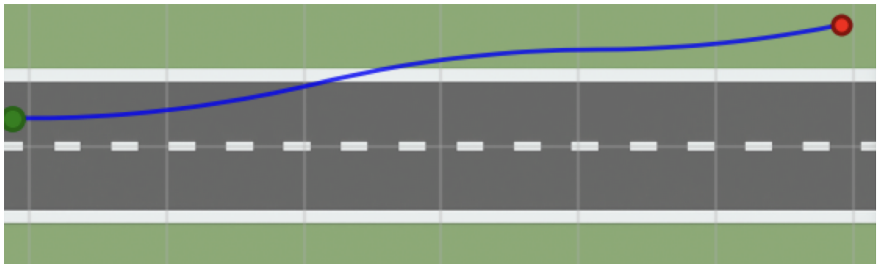
Abbildung 39: Trajektorie bei 1,0 m/s Seitenwind mit erhöhten Balance-Gains: stabilisierte Fahrt ohne Umkippen; die Abdrift wird begrenzt und anschließend abgebaut.
