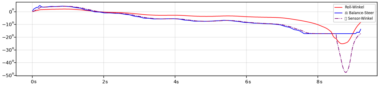
Abbildung 38: Zeitverlauf bei 1,0 m/s (Baseline-Regler): ansteigende Rollauslenkung und instabiles Verhalten nach \approx 7 s. X-Achse: Zeit in Sekunden, Y-Achse: Winkel in Grad
