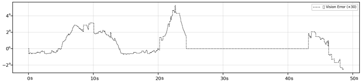
Abbildung 30: S-Kurve: visionbasierter Querfehler \tilde{e}_y
