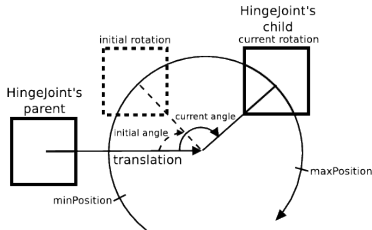
Abbildung 7: Aktuatoren im Fahrradmodell.
