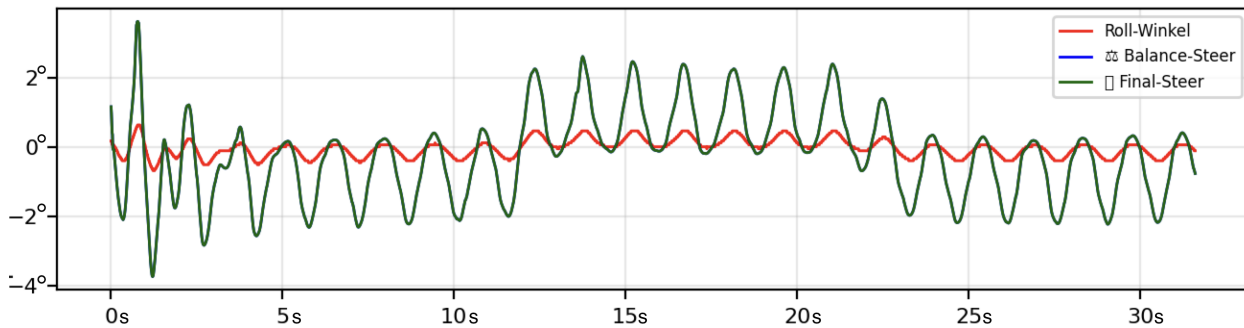
Abbildung 40: Zeitreihen bei 1,0 m/s mit erhöhten Gains: gedämpfter Rollwinkelverlauf; höhere, aber tolerierbare Lenkaktivität (keine Sättigung, keine Divergenz). X-Achse: Zeit in Sekunden, Y-Achse: Winkel in Grad
