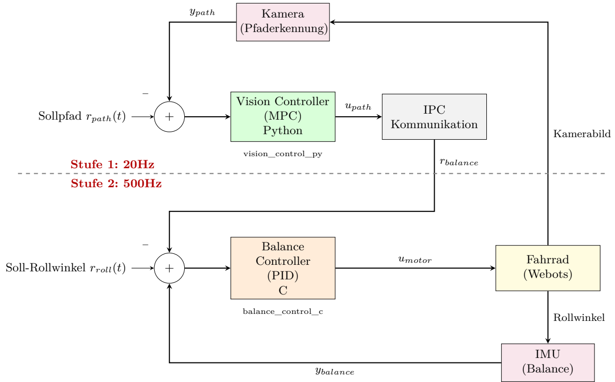
Abbildung 10: Zweistufige Kaskadenregelung: Vision-MPC (Stufe 1) für Spurführung und Balance-PID (Stufe 2) für Stabilisierung
