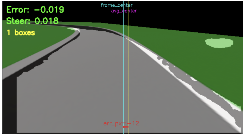
Abbildung 11: YOLOv8-Segmentierung.
