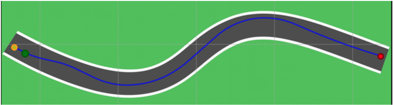
Abbildung 31: S-Kurve mit ROI-Regler
