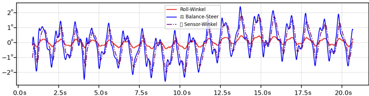
Abbildung 49: Zeitverläufe mit angepasstem Balance PID (Fall D, M = 2,0\text{ m} ). X-Achse: Zeit in Sekunden, Y-Achse: Winkel in Grad
