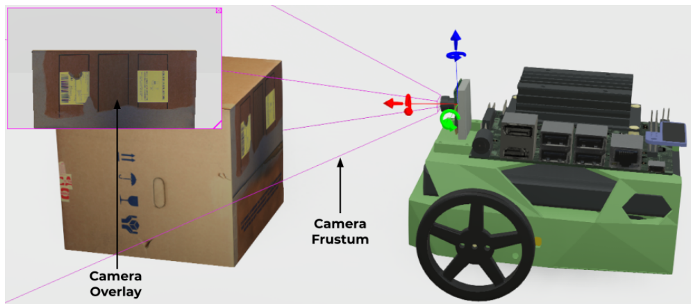
Abbildung 4: Kamera-Knoten in Webots.
