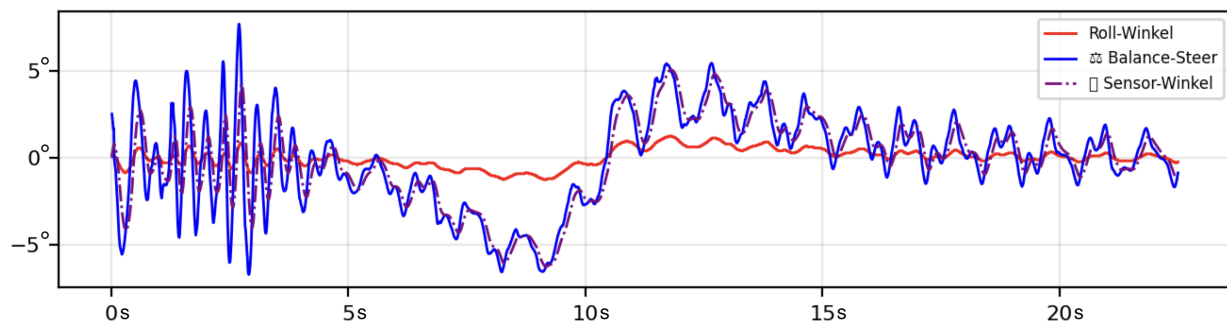
Abbildung 51: Zeitverläufe mit angepasstem Balance PID (Fall E, M = 4,0\text{ m} ). X-Achse: Zeit in Sekunden, Y-Achse: Winkel in Grad
