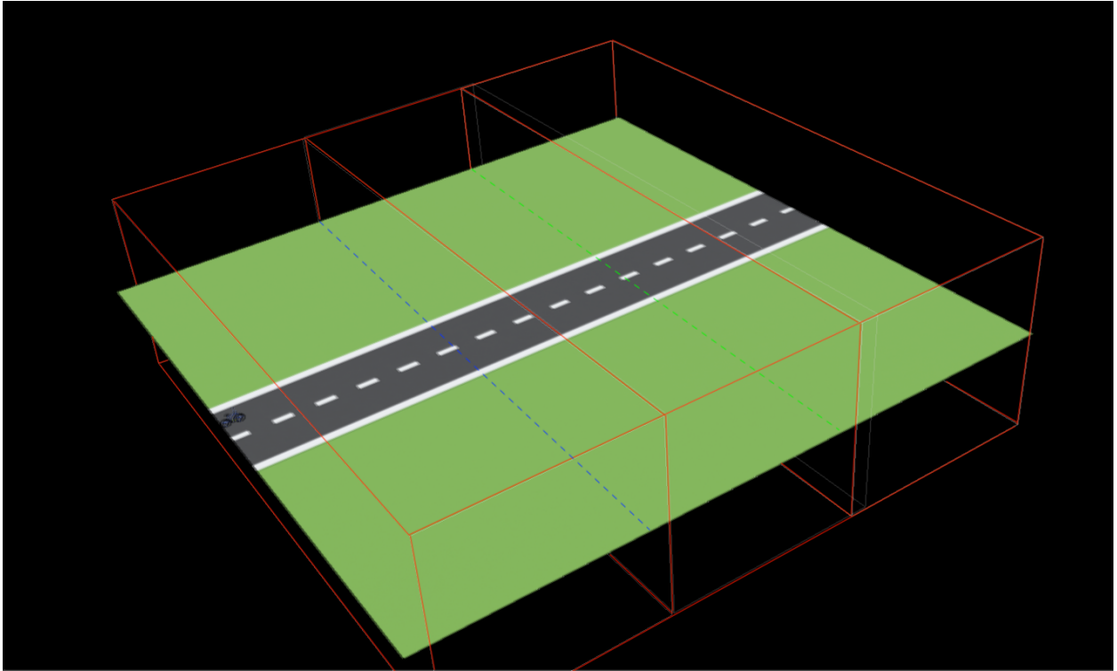
Abbildung 34: Versuchsaufbau: Gerade Strecke mit drei seitlichen Windkanälen (rote Drahtgitterboxen). Die Fahrbahnmitte dient als Referenz für die Spurführung.
