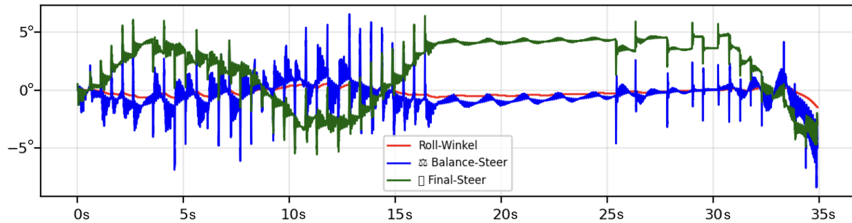
Abbildung 17: Kurvenfahrt mit PID-Regler und YOLO-Spurführung. X-Achse: Zeit in Sekunden, Y-Achse: Winkel in Grad
