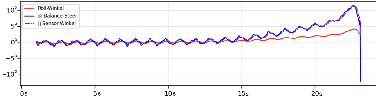
Abbildung 45: Zeitverläufe Rollwinkel/Balancelenkung (Fall B, M = 2,0 m, Baseline-Gewichte). X-Achse: Zeit in Sekunden, Y-Achse: Winkel in Grad
