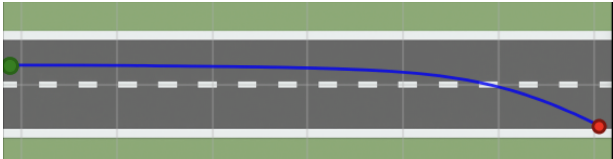
Abbildung 46: Trajektorie mit retuntem Balance-PID (Fall B, M = 2,0 m).
