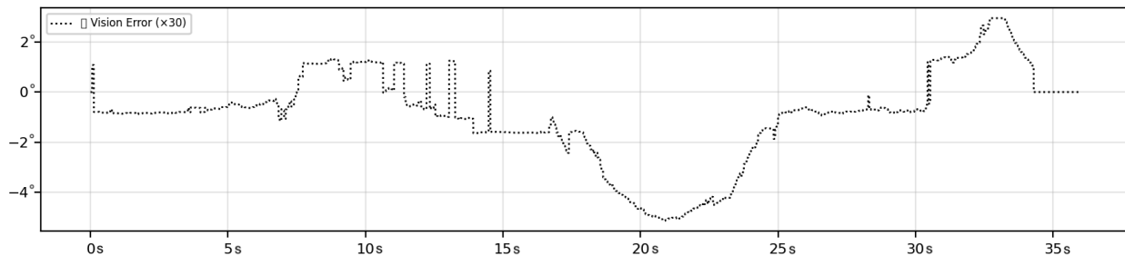
Abbildung 18: ROI-Querfehler während der PID-Regler-Fahrt (YOLO)
