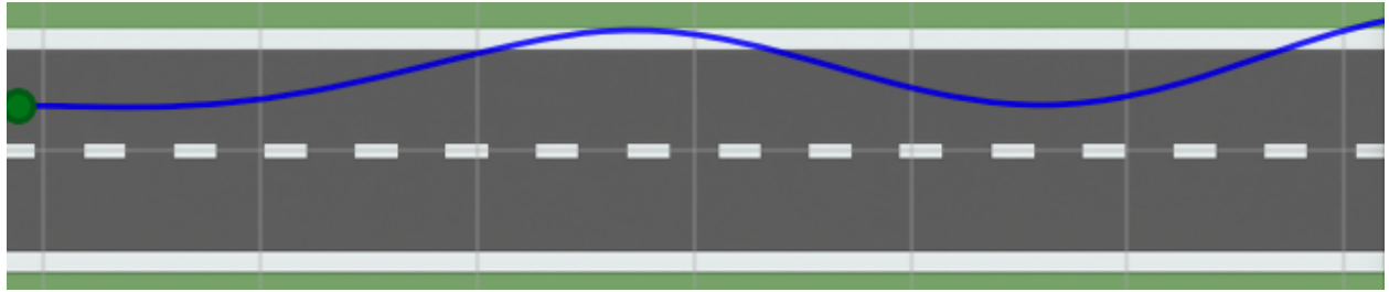
Abbildung 35: Trajektorie bei 0,5 m/s Seitenwind: Blaue Linie = Fahrzeugspur; Start (grün) und Endpunkt (rot). Die Auslenkung in den ersten beiden Windsegmenten wird nach dem dritten Segment wieder abgebaut.
