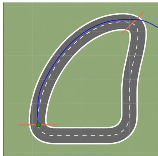
Abbildung 23: Gefahrene Trajektorie (PID-Regler, ROI)
