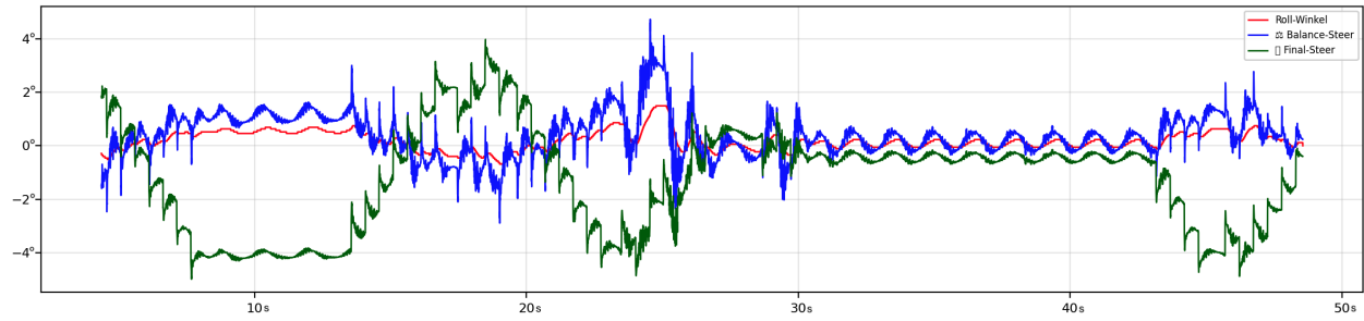
Abbildung 29: S-Kurve: ausgewählte Zeitreihen (Rollwinkel, Balance-Soll, final_steer ). X-Achse: Zeit in Sekunden, Y-Achse: Winkel in Grad
