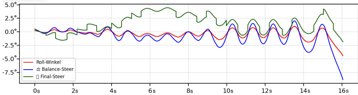
Abbildung 14: Kurvenfahrt mit reinem P-Regler (Zeitreihen). X-Achse: Zeit in Sekunden, Y-Achse: Winkel in Grad
