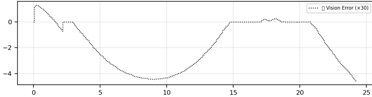
Abbildung 25: ROI-Querfehler während der P-Regler-Fahrt (Vision)
