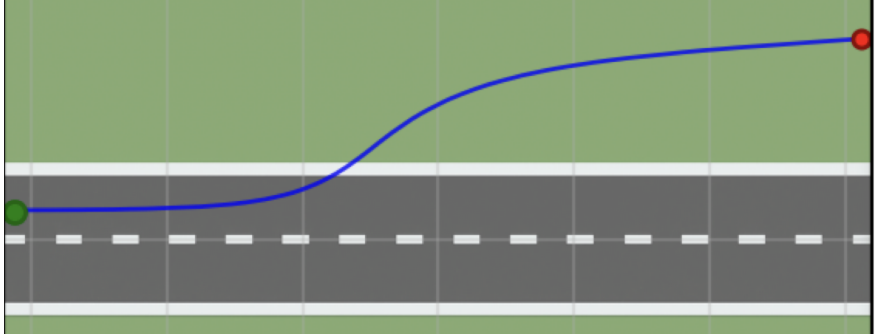
Abbildung 50: Trajektorie durch den Hügel (Fall E, M = 4,0\text{ m} ).
