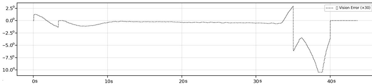
Abbildung 22: ROI-Querfehler während der PID-Regler-Fahrt (ROI)
