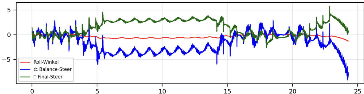
Abbildung 24: Kurvenfahrt mit P-Regler (Vision) und PID-Regler (Balance). X-Achse: Zeit in Sekunden, Y-Achse: Winkel in Grad
