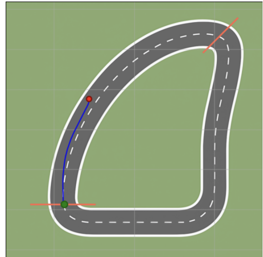
Abbildung 16: Gefahrene Trajektorie (P-Regler)
