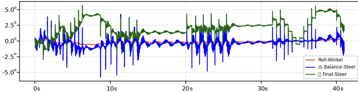
Abbildung 21: Kurvenfahrt mit PID-Regler und ROI-Fallback-Erkennung. X-Achse: Zeit in Sekunden, Y-Achse: Winkel in Grad
