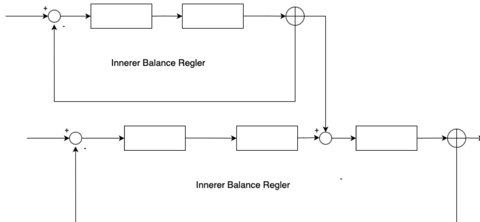
Figure 10: Kombimierter Regler.
