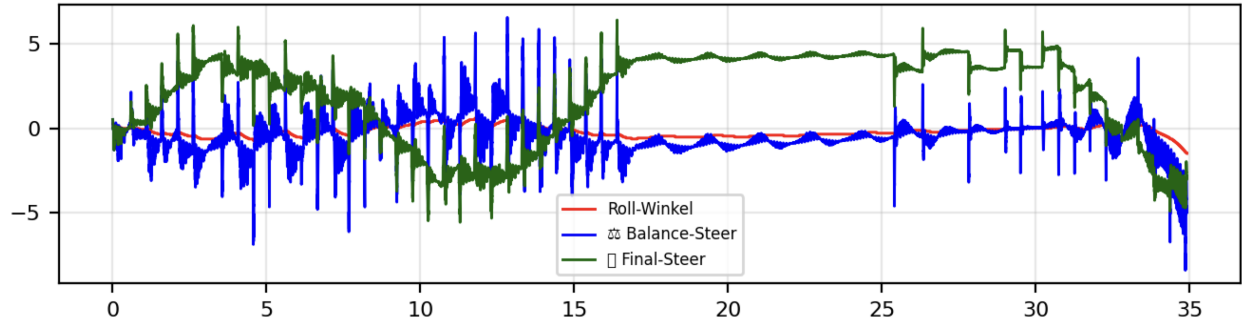
Figure 20: Kurvenfahrt mit PID-Regler und YOLO-Spurführung
