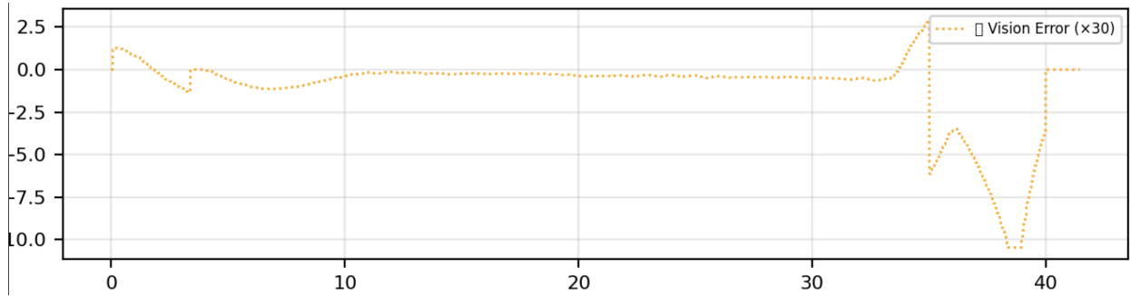
Figure 25: ROI-Querfehler während der PID-Regler-Fahrt (ROI)
