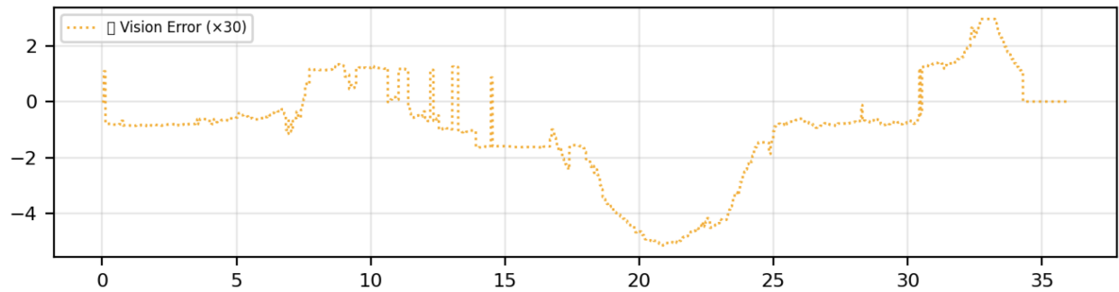
Figure 21: ROI-Querfehler während der PID-Regler-Fahrt (YOLO)
