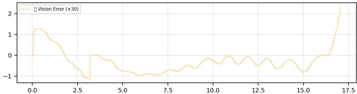
Figure 19: ROI-Querfehler während der P-Regler-Fahrt
