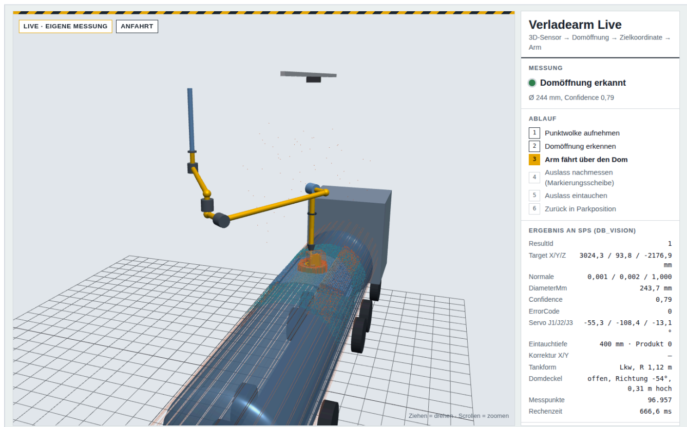
Bild 2: Live-Ansicht (Browser) mit simuliertem Tankwagen: Punktwolke, erkannte Domöffnung (Ø 244 mm), offener Deckel, geplante Armbewegung und die an die SPS übergebenen Werte.
