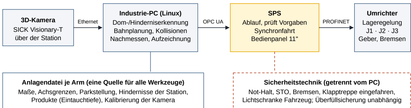
Bild 1: Aufgabenteilung. Der PC plant, die SPS prüft und fährt, die Sicherheitstechnik wirkt unabhängig vom PC.
