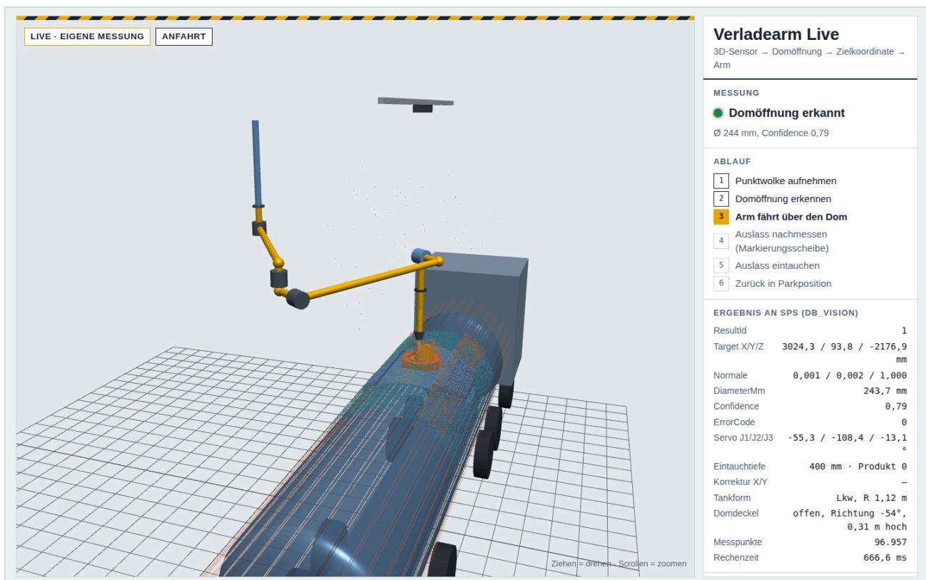
Bild 2: Live-Ansicht (Browser) mit simuliertem Tankwagen: Punktwolke, erkannte Domöffnung (Ø 244 mm), offener Deckel, geplante Armbewegung und die an die SPS übergebenen Werte.
