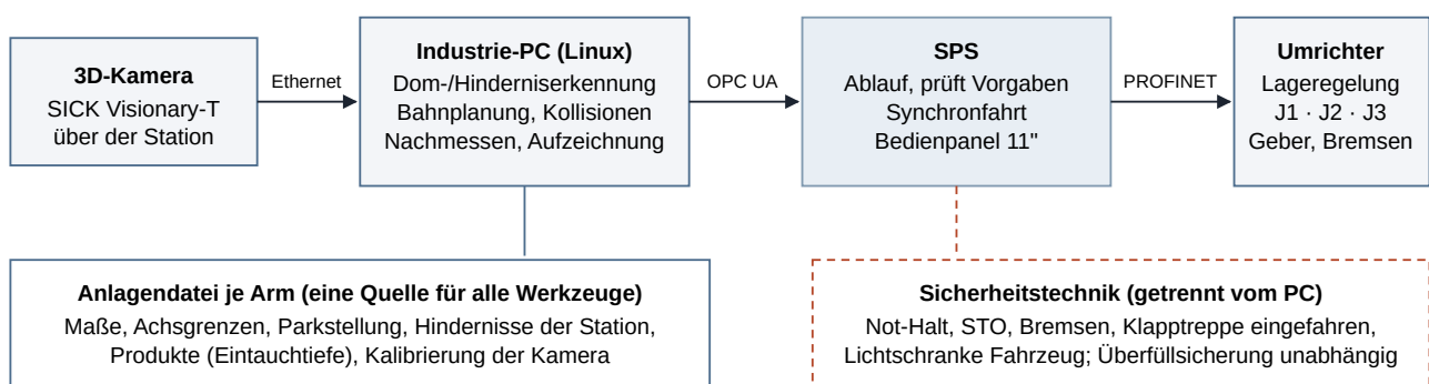
Bild 1: Aufgabenteilung. Der PC plant, die SPS prüft und fährt, die Sicherheitstechnik wirkt unabhängig vom PC.
