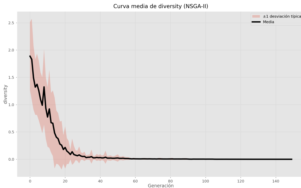
Figura 17: Diagrama de diversidad de los Frentes de Pareto.
