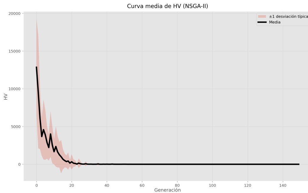
Figura 16: Diagrama del hipervolumen de los Frentes de Pareto.
