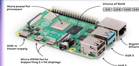
Raspberry Pi 4B de 8GB RAM
