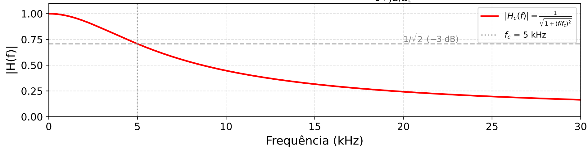
Espectro do Sinal — Agudos Atenuados pelo Cabo
