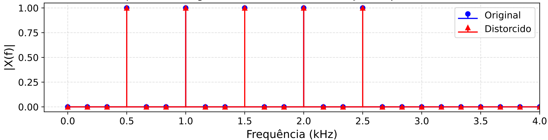
Espectro de Magnitude — IDÊNTICO! (distorção é apenas na fase)
