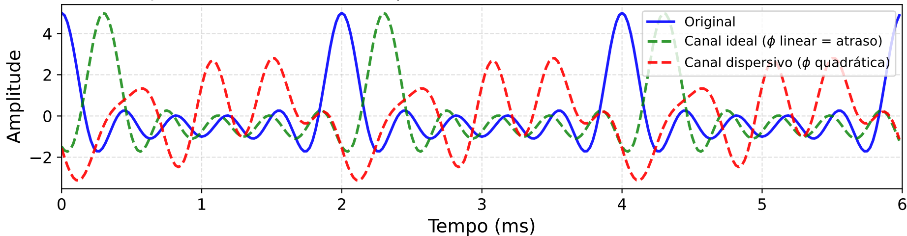
Distorção de Fase — Mesmas amplitudes, fases diferentes → forma de onda alterada
